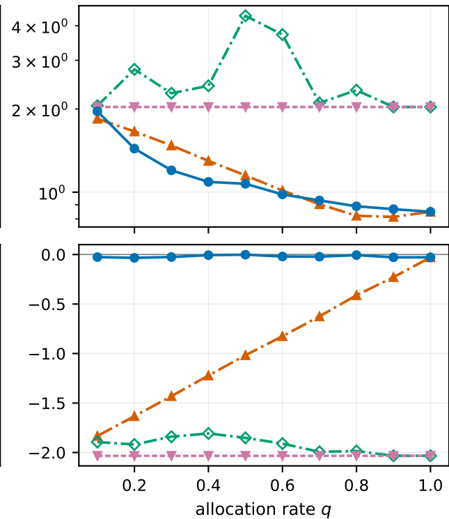
MovieLens
