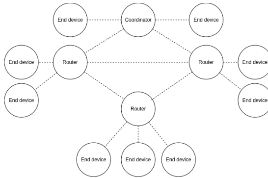
Hình 2.2: Mesh topology – Định tuyến đa chặng linh hoạt
