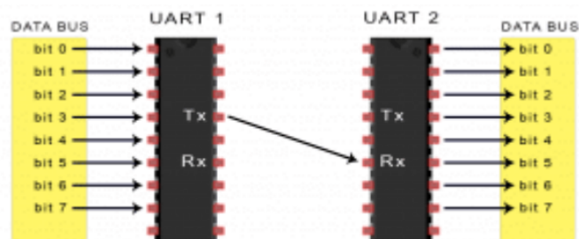
Hình 2.7: Kết nối UART vật lý giữa Host và NCP
