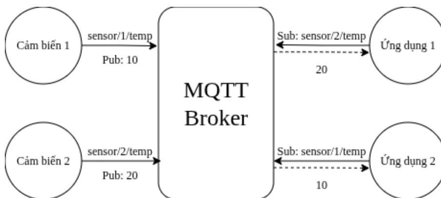
Hình 2.6: Kiến trúc truyền thông Publish/Subscribe qua Broker trung gian
