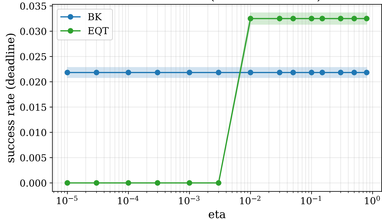
Success vs eta (extended <0.01 )
