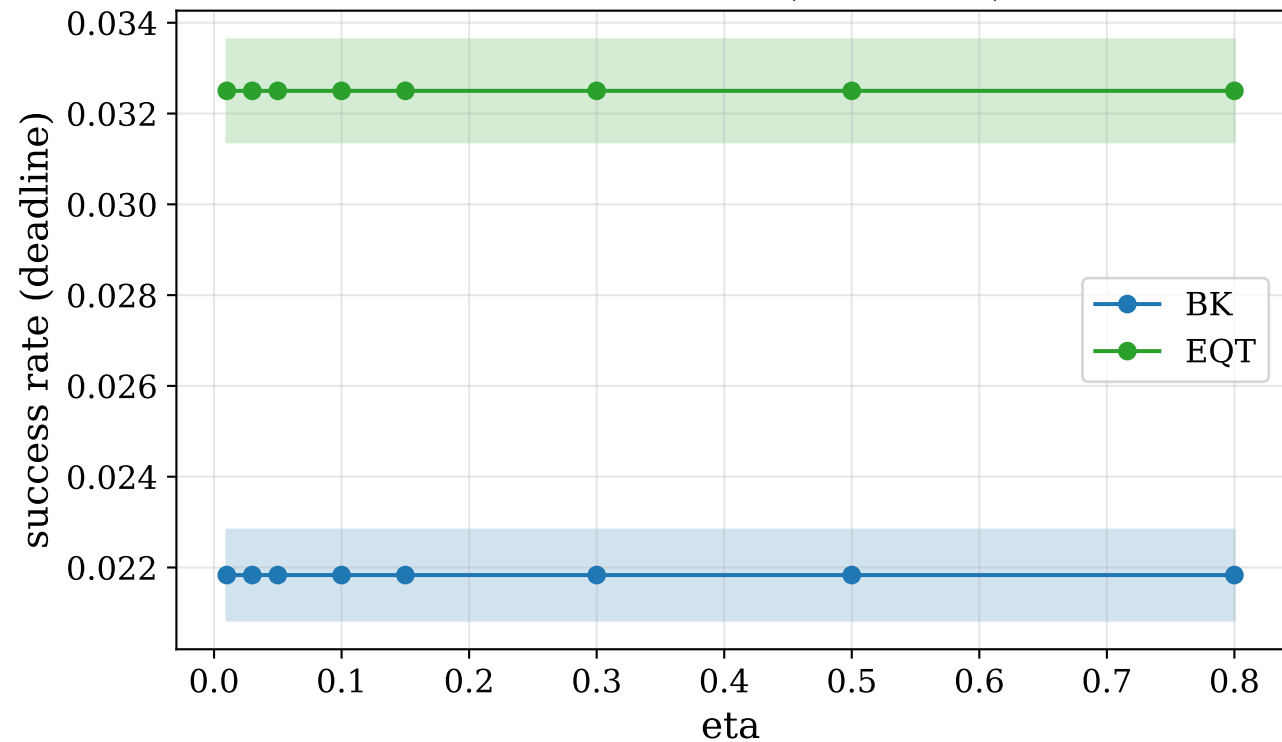
Success vs eta (NSFNET)
