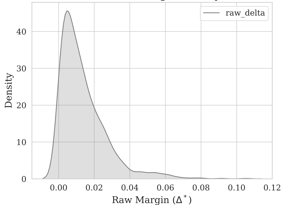
Raw DPO Margin Density
