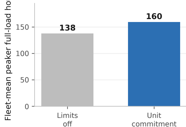
(b) Peaker utilisation, 2050
