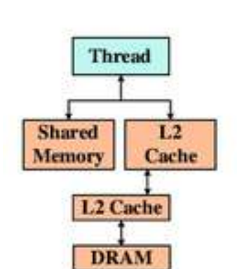
(b) Fermi Mem. Hierarchy
