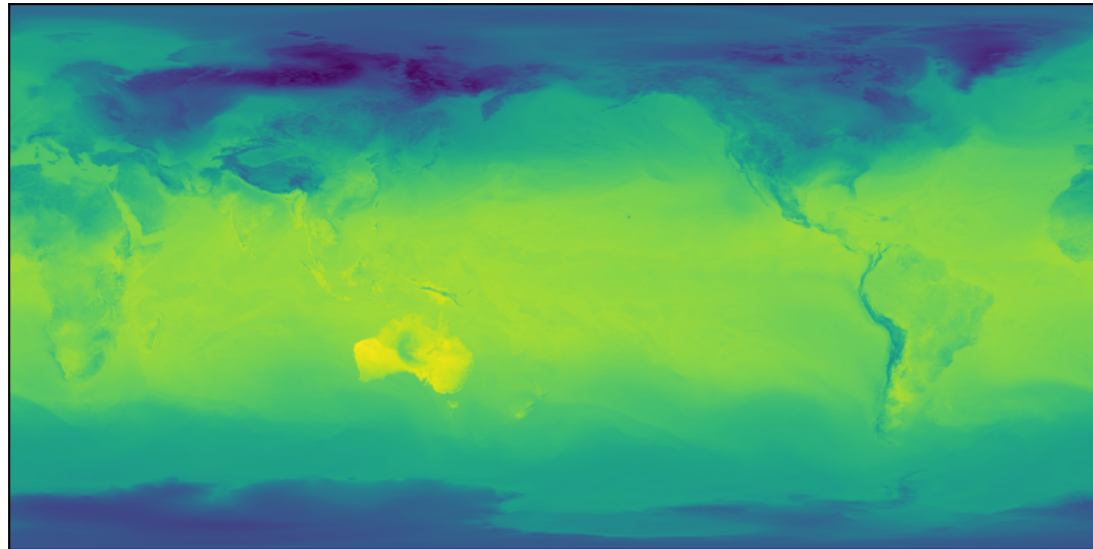
ERA5
