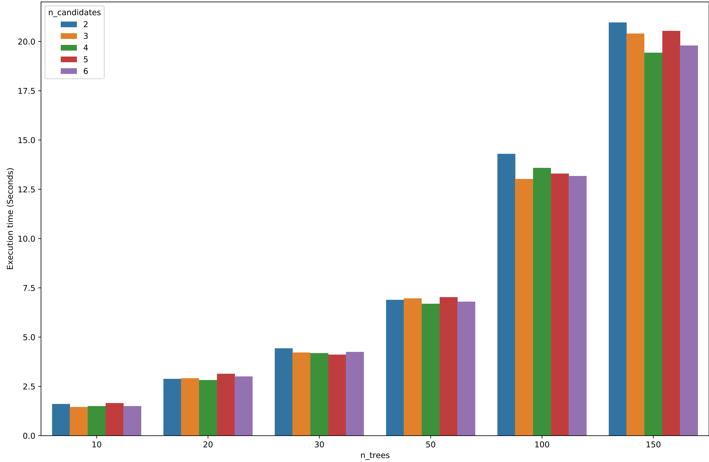
ItalyPowerDemand
