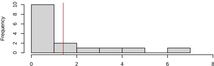
n = 16
