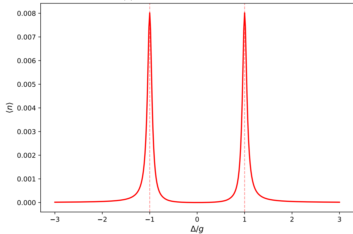
(d) Vacuum Rabi doublet in transmission
