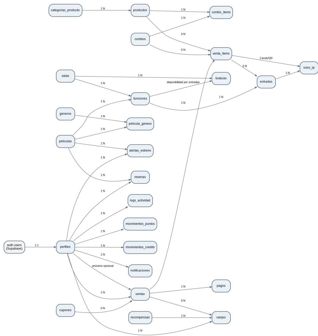
Figura 1 - Relación conceptual propuesta. Algunas relaciones operativas se resuelven a través de claves y consultas, no como relaciones directas entre todas las tablas.
