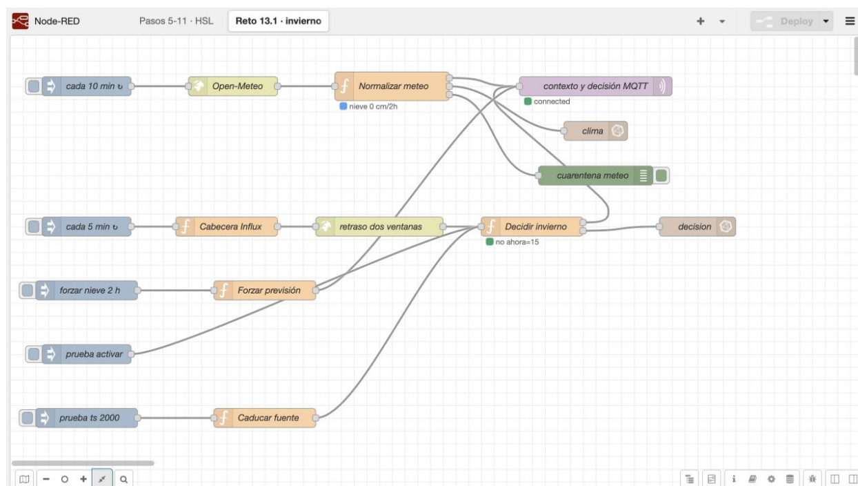
Figura 7. Flujo de adquisición meteorológica y decisión por ventanas. Captura del laboratorio.
