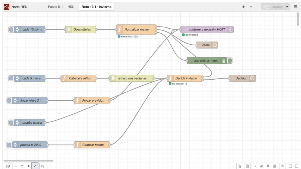
Figura 7. Flujo de adquisición meteorológica y decisión por ventanas. Captura del laboratorio.
