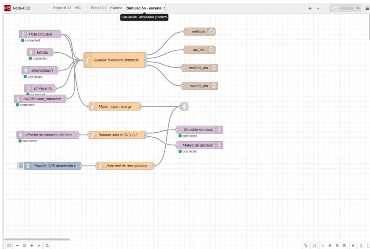
Figura 18. Flujo de almacenamiento, mapa y protección de la retención en Node-RED
