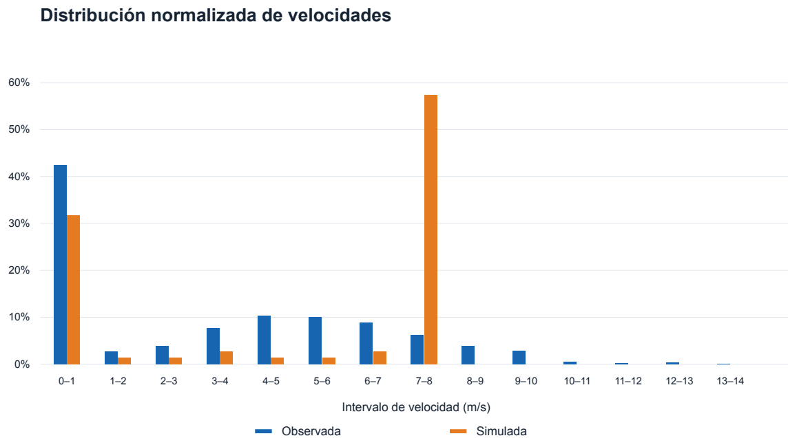
Figura 16. Distribuciones de velocidad real y simulada, en porcentajes
