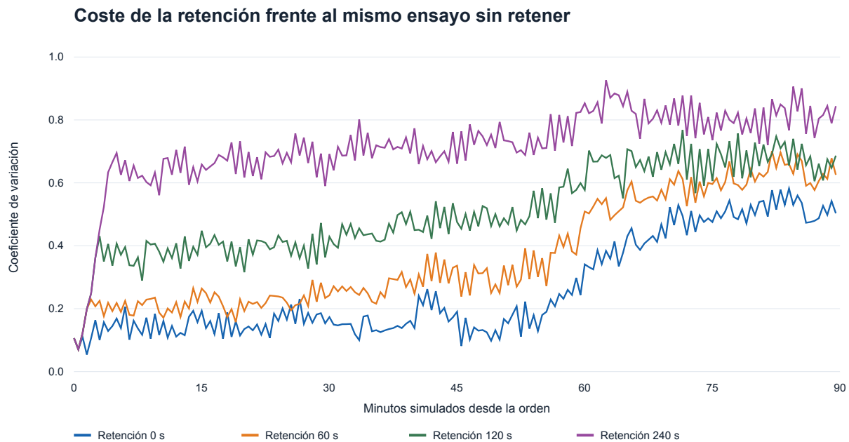
Figura 19. Ensayos pareados de retención y control sin intervención
