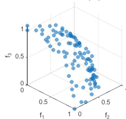
MOPSO-FM (F5)
