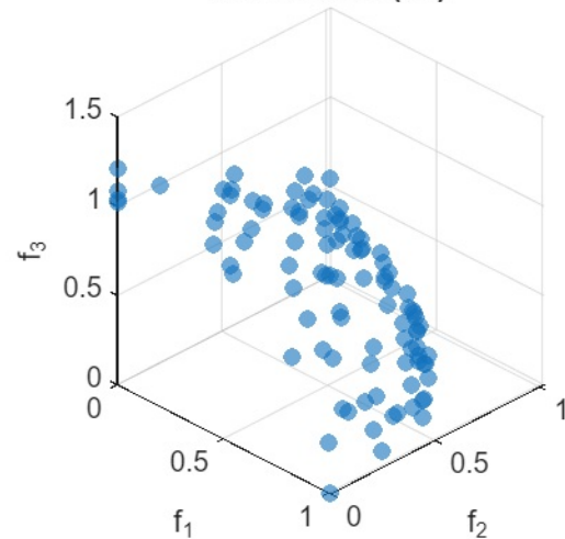
MOPSO-CD (F5)
