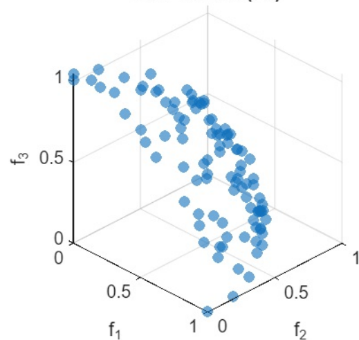
MOPSO-ML (F5)
