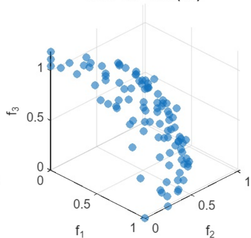
MOPSO-Grid (F5)
