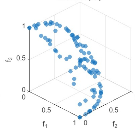
MOABC (F5)
