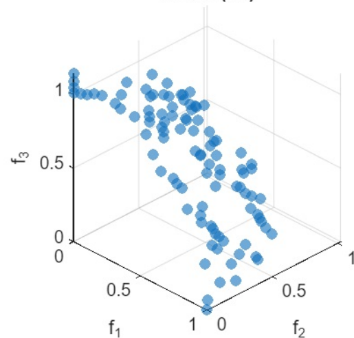
MOFA (F5)
