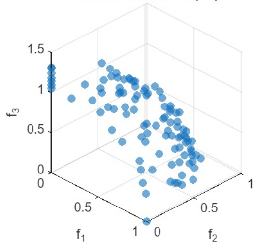
Classical-MOPSO (F5)
