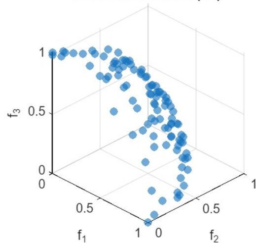
SA-MOPSO-FVML (F5)
