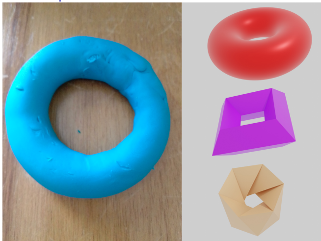
FIG. 3 : Tores topologiques
