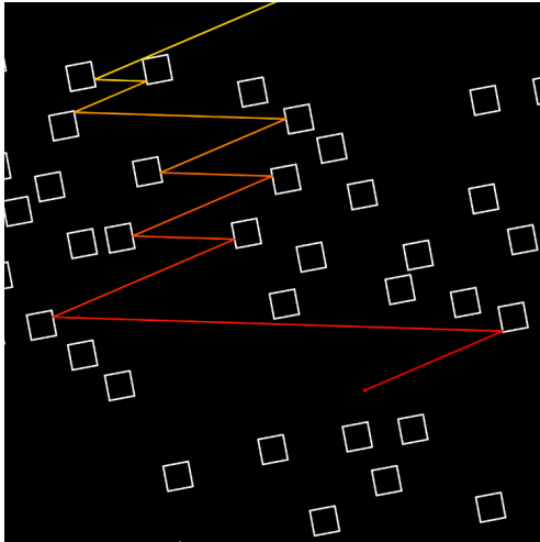
FIG. 9 : Dynamique du wind tree, par Antonsen
