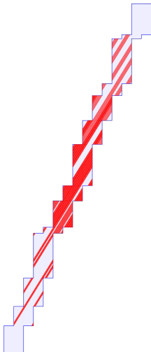
FIG. 8 : Escalier à hauteur variable
