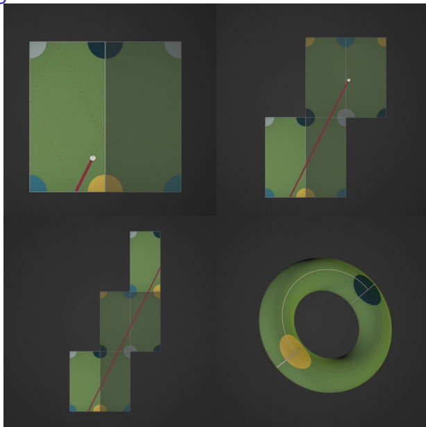
FIG. 4 : Dépliage d'une trajectoire de billard sur une table rectangulaire
