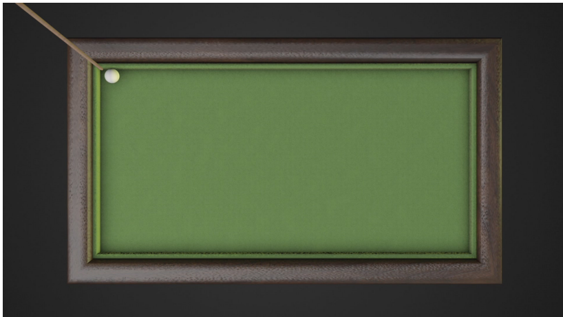
FIG. 3 : Départ d'une trajectoire de billard sur une table rectangulaire
