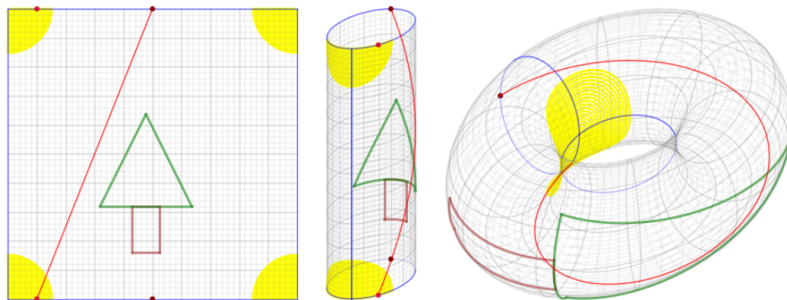
FIG. 2 : Trajectoire sur le tore, par Lelièvre et Goujard
