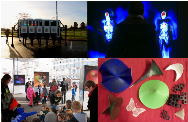
FIG. 10 : La chambre de Lorentz, Première intimité de l'être, une exposition Imaginary, objets mathématiques imprimés en 3D
