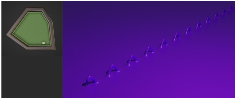
FIG. 6 : Billard irrationnel par Hale, monstre du Loch Ness par MS.
