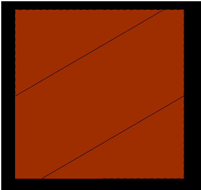
Figure 9: On obtient le flot sur le tore
