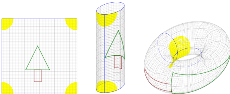
Figure 3: Quelques dessins pour comprendre le tore plat par Lelièvre et Goujard.
