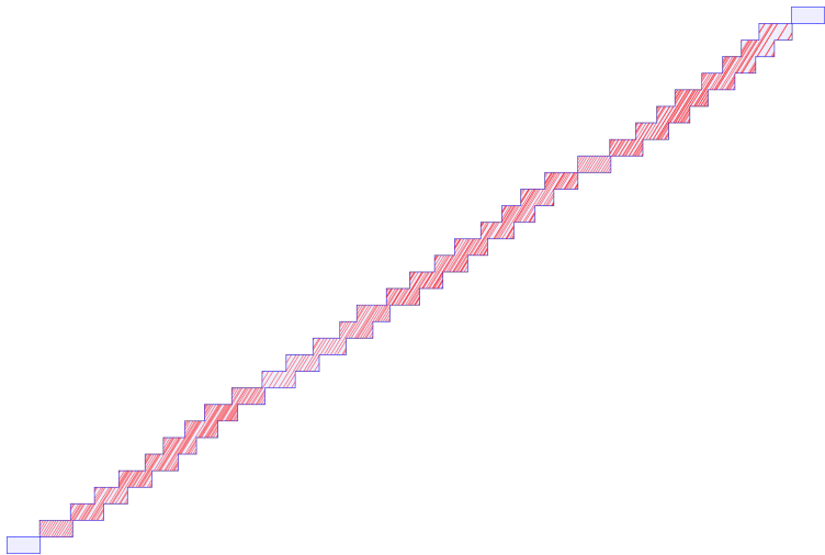
Figure 14: Escalier à recollement variable
