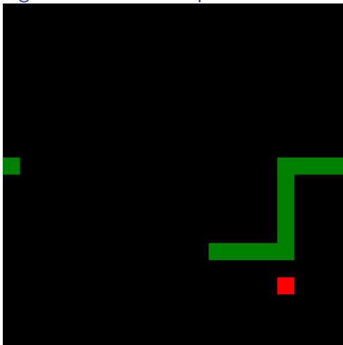
Figure 6: Tableau du jeu du serpent sur un tore, par Primož Žnidar
