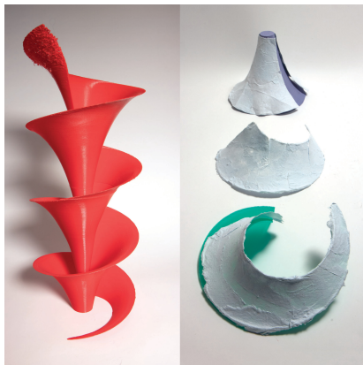
Figure 21: Papier hyperbolique par Abrams, Paul et MS, photos par Harris.
