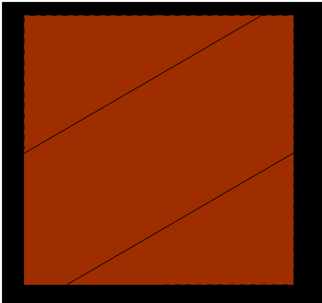
Figure 12: On obtient le flot sur le tore
