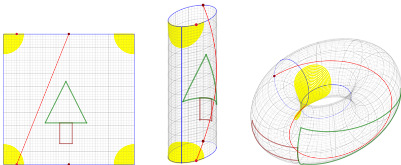
Figure 7: Trajectoire sur le tore, par Lelièvre et Goujard.
