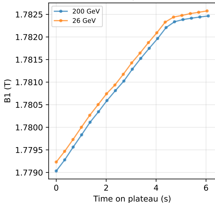
SFTPRO top — B1 (T)
