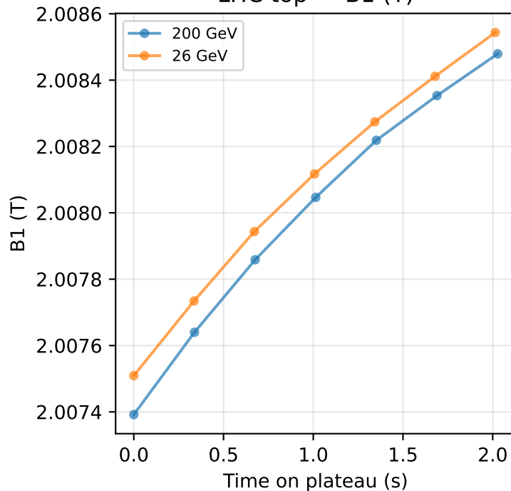
LHC top — B1 (T)
