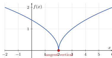
Figura 2.28. Interpretació gràfica de la continuïtat i la no derivabilitat a x = 2 .
