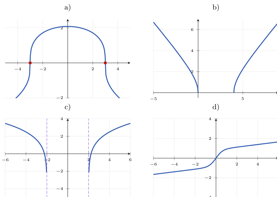
Figura 2.34. Representacions dels apartats a-d de l'exercici 2.22.
