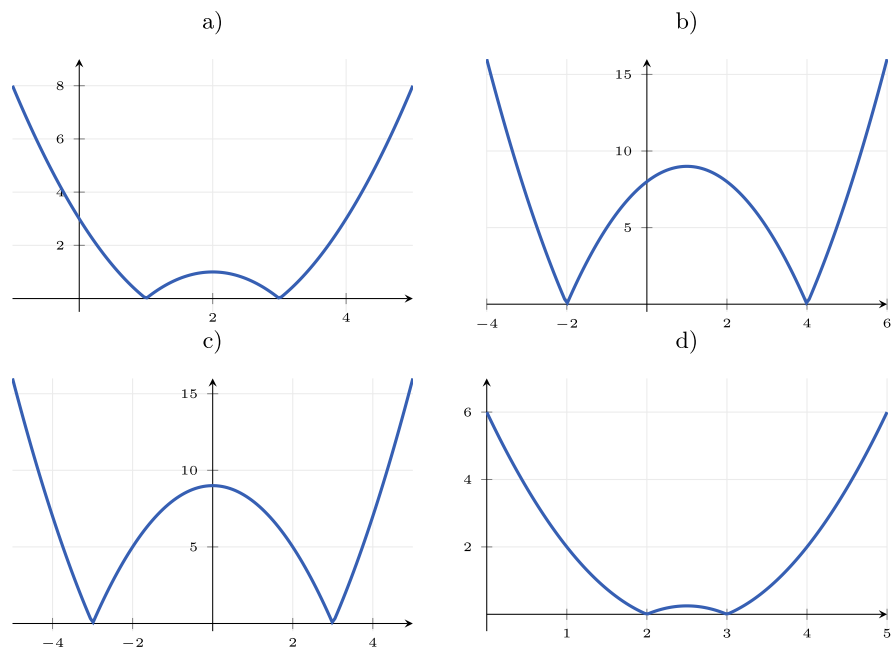
Figura 2.37. Representacions de les funcions de l'exercici 2.24.
