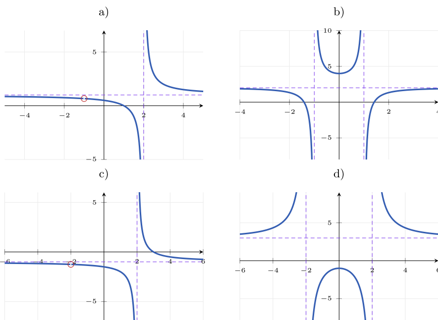
Figura 2.31. Representacions dels apartats a-d de l'exercici 2.19.
