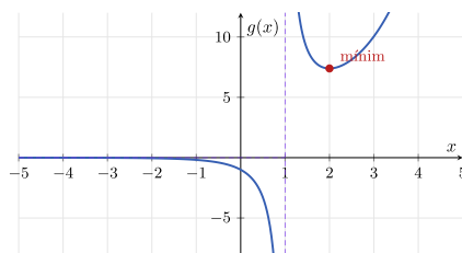
Figura 2.39. Representació completa de la funció de l'exercici 2.27.
