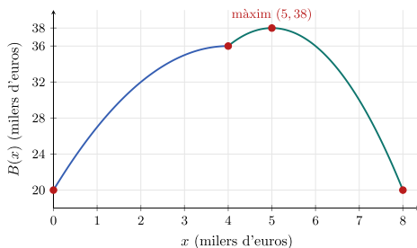
Figura 2.41. Representació del benefici de l'exercici 2.37.
