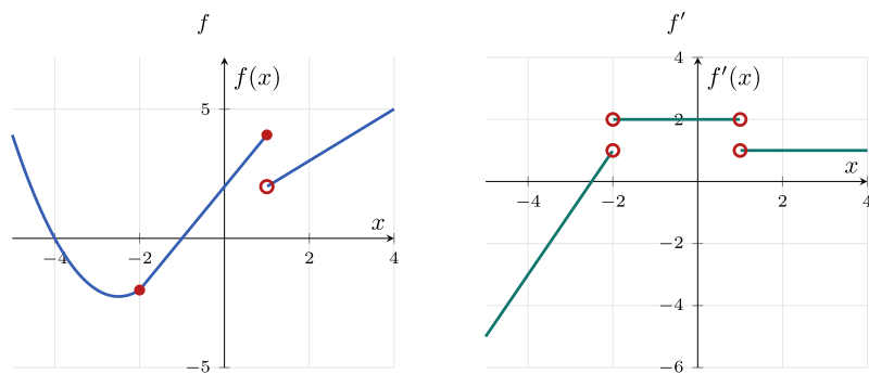
Figura 2.29. Representació de f i de f' en l'exercici 2.6.
