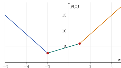
Figura 2.40. Representació de la funció de l'exercici 2.28.
