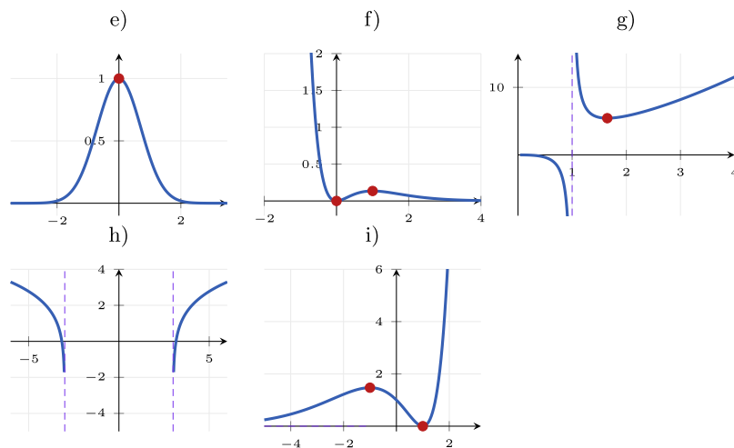
Figura 2.35. Representacions dels apartats e-i de l'exercici 2.22.
