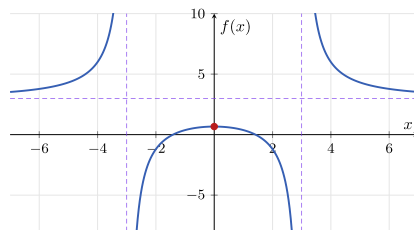
Figura 2.38. Representació completa de la funció de l'exercici 2.26.
