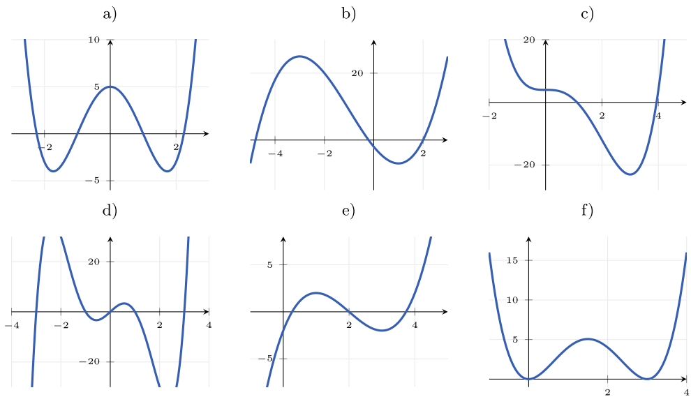
Figura 2.30. Representacions de les funcions polinòmiques de l'exercici 2.18.
