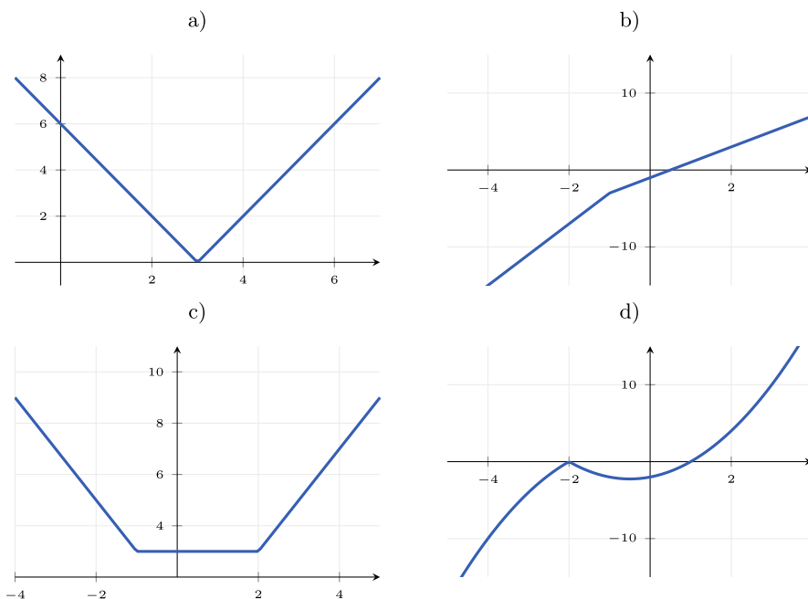
Figura 2.36. Representacions de les funcions de l'exercici 2.23.
