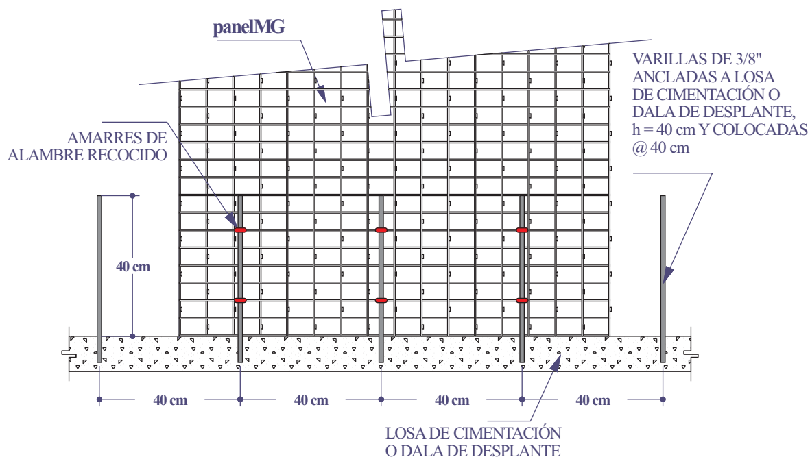
ANCLAJE DE MUROS sin escala
