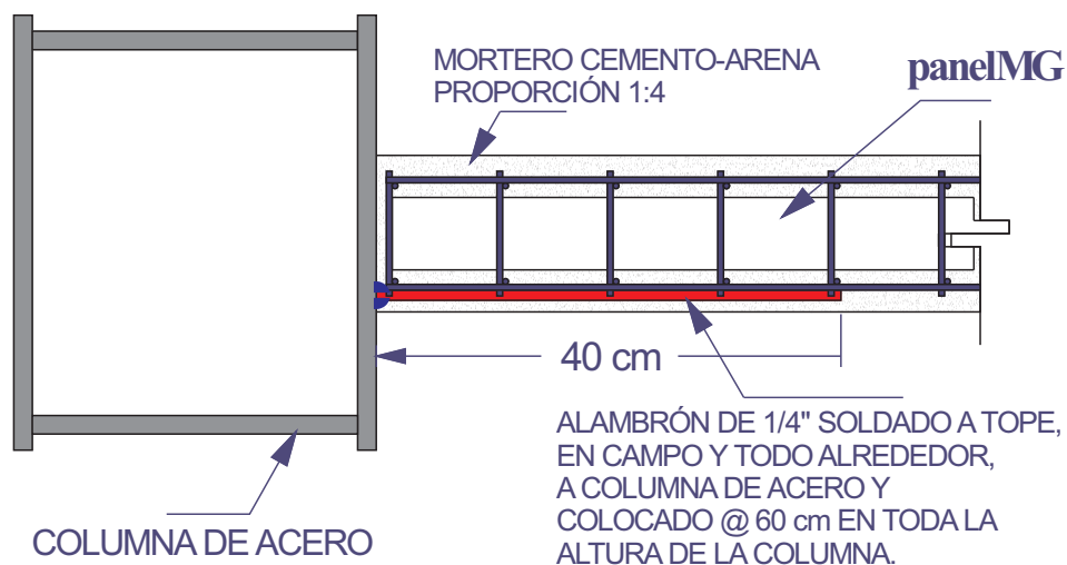
ANCLAJE DE MURO DIVISORIO A COLUMNA DE ACERO sin escala
