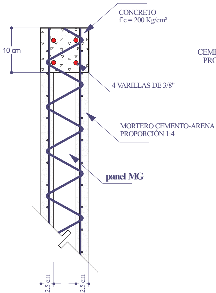
DALA DE CORONACIÓN INTEGRADA AL PANEL sin escala
