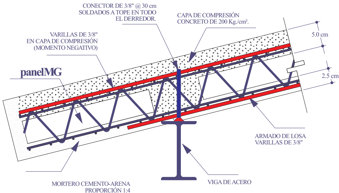
APOYO DE LOSA INCLINADA EN VIGA DE ACERO
