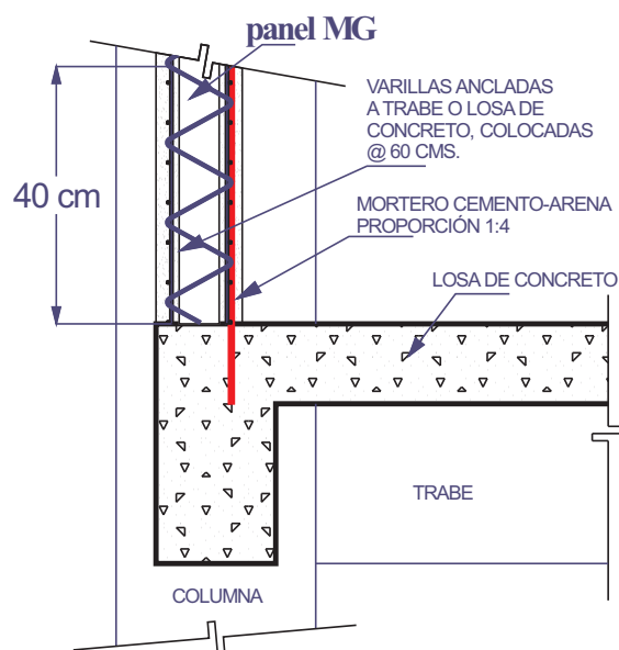
ANCLAJE DE MURO DIVISORIO A ESTRUCTURA DE CONCRETO CON ANCLAS DE VARILLAS sin escala
