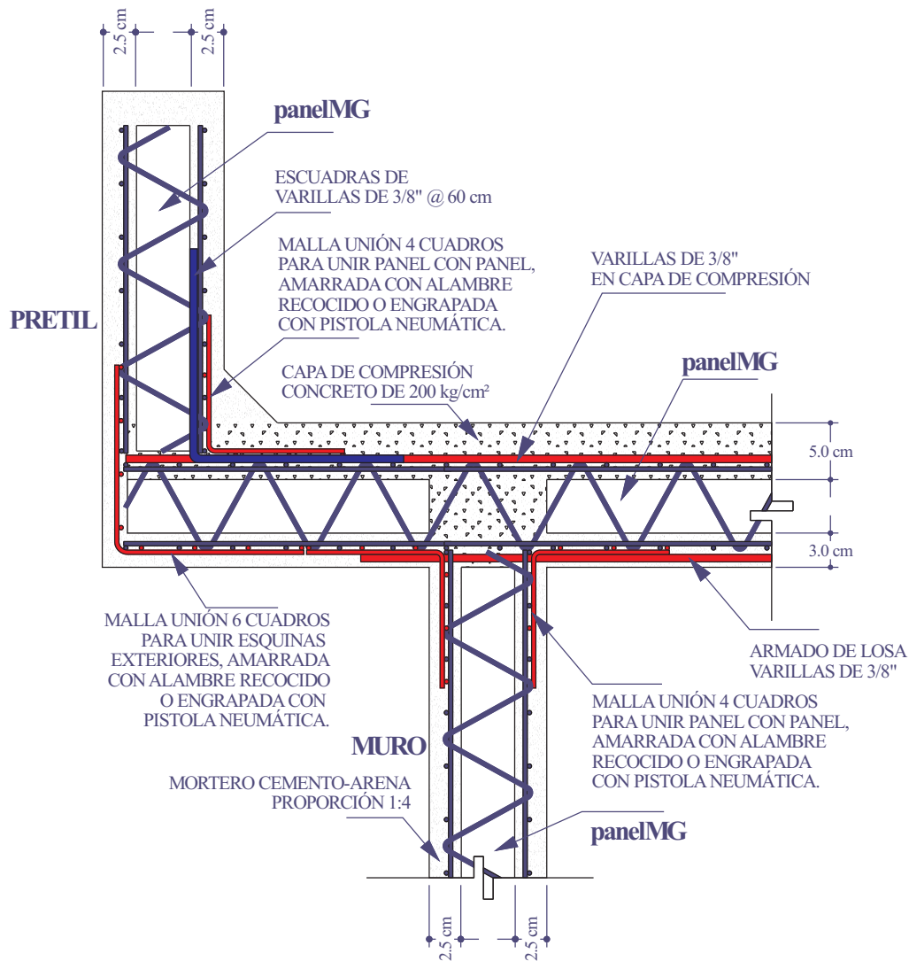
UNIÓN DE MURO CON VOLADIZO Y PRETIL sin escala
