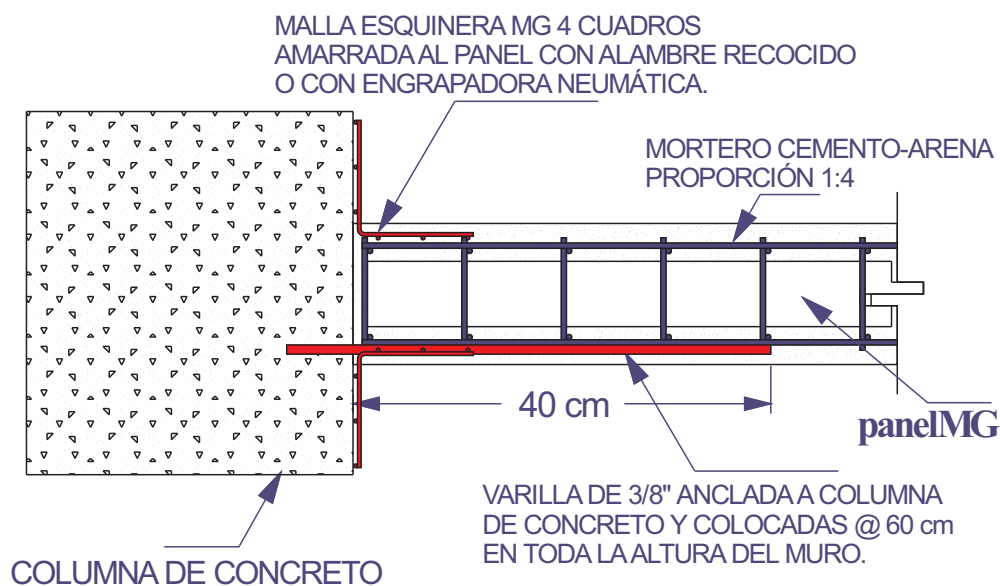
ANCLAJE DE MURO A COLUMNA DE CONCRETO sin escala
