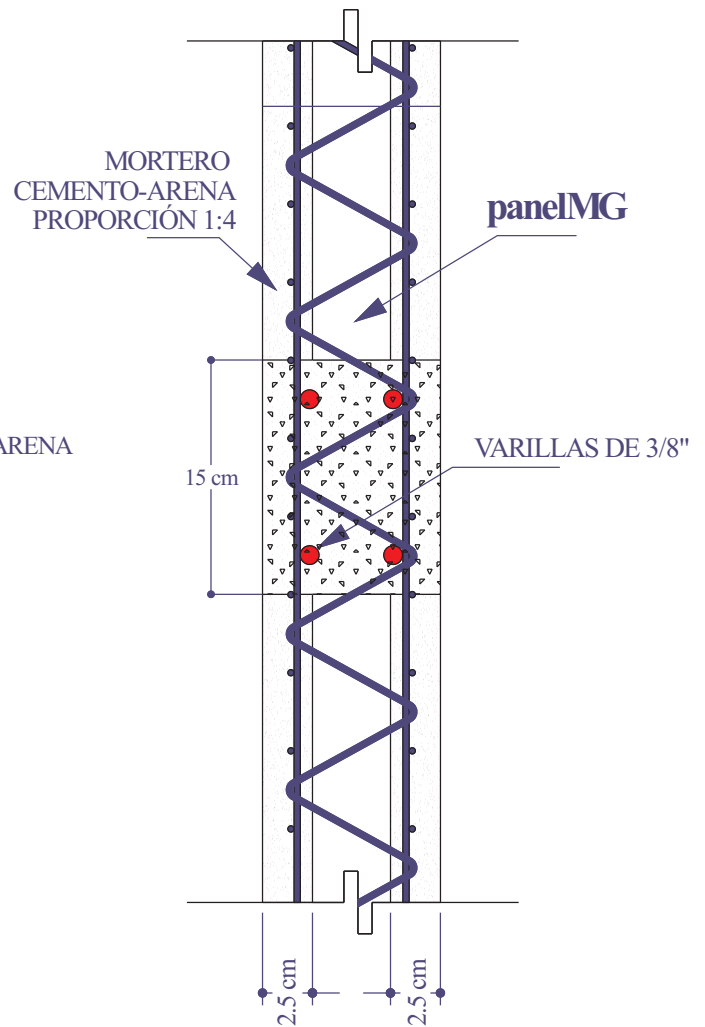
DALA INTEGRADA AL MURO DE PANEL sin escala
