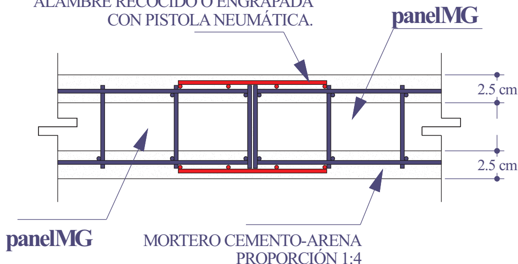
UNIÓN DE PANEL CON PANEL (muros) sin escala
