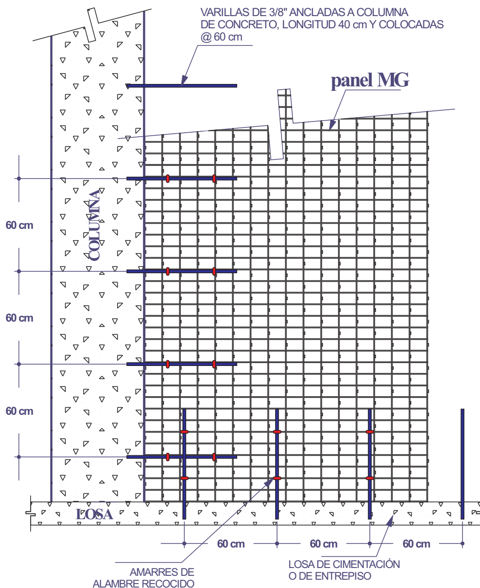
ANCLAJE DE MUROS DIVISORIOS A COLUMNA DE CONCRETO sin escala
