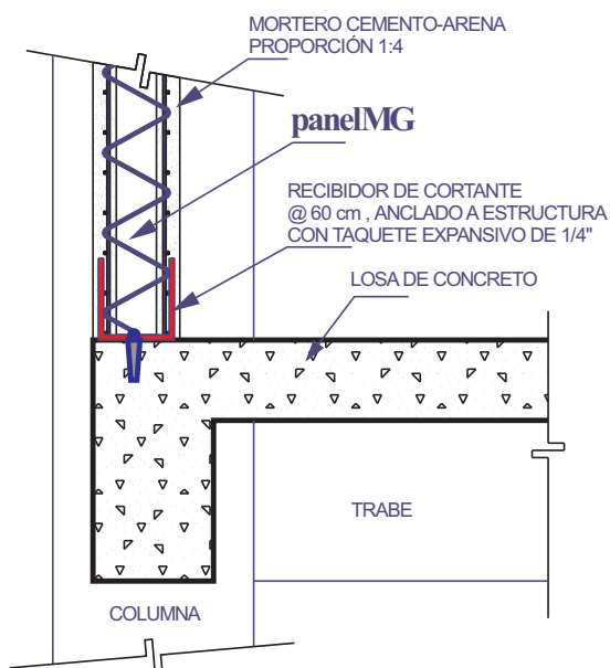
ANCLAJE DE MURO DIVISORIO A ESTRUCTURA DE CONCRETO CON RECIBIDOR DE CORTANTE sin escala
