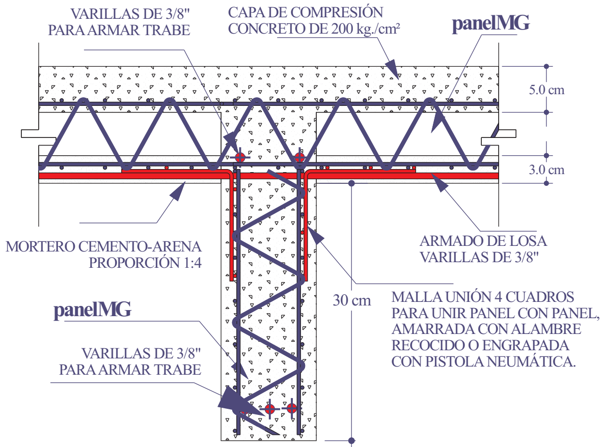
TRABE "T2" INTEGRADA AL PANEL sin escala
