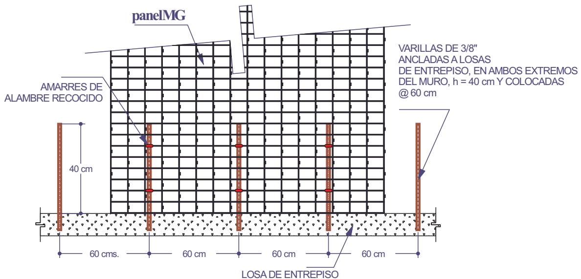
ANCLAJE DE MUROS DE FACHADA sin escala
