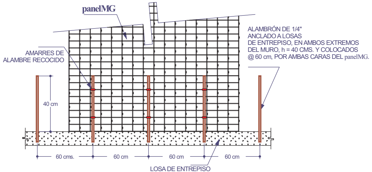
ANCLAJE DE MUROS INTERIORES sin escala
