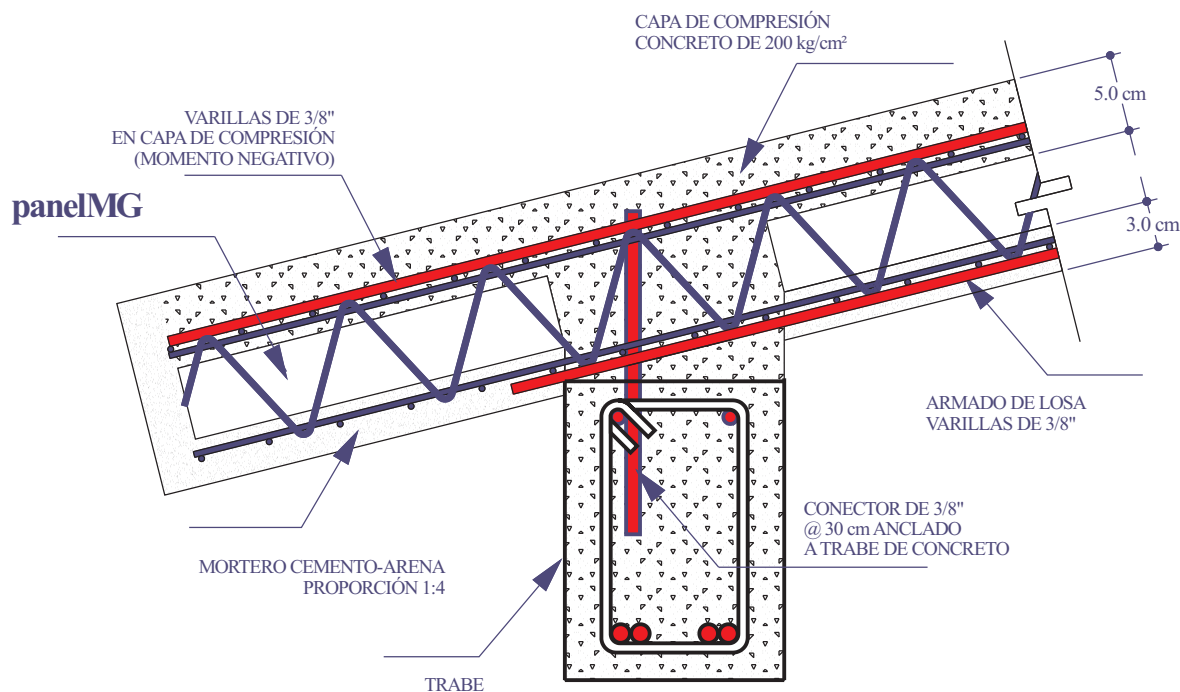
ANCLAJE A TRABE DE CONCRETO sin escala
