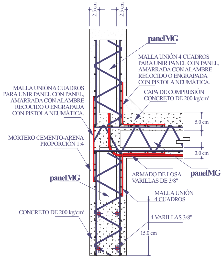
CERRAMIENTO "C1" sin escala
