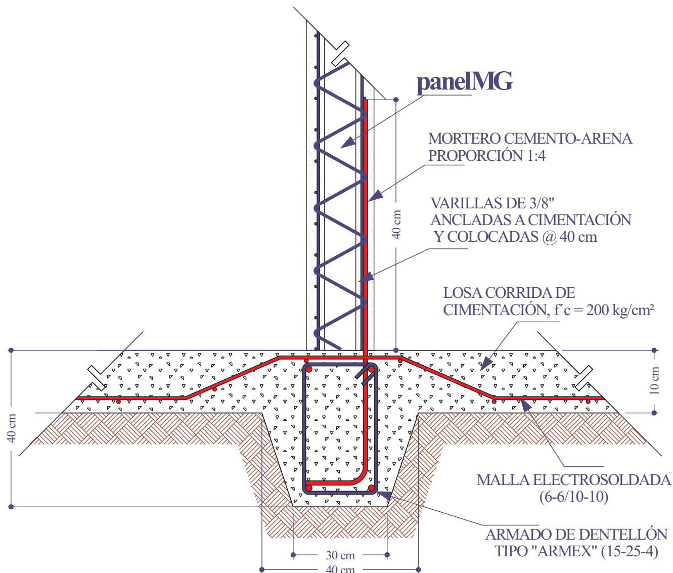
ANCLAJE DE MURO INTERIOR A LOSA DE CIMENTACIÓN sin escala
