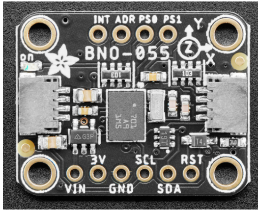
Figura 2.17: BNO055 Bosch Sensortec. Configurazione dei pin e breakout board
