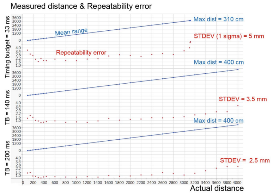
Figura 2.22: VL53L1X, prestazioni di misura
