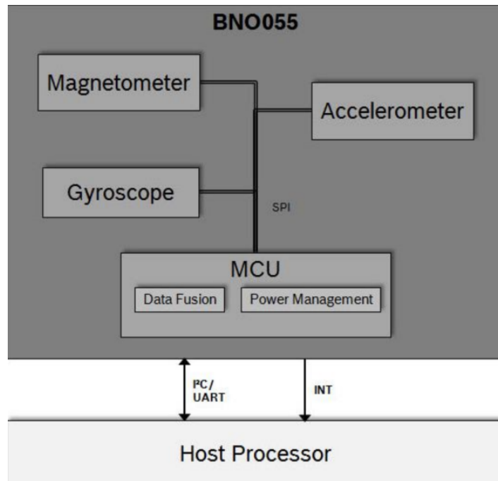
Figura 2.18: BNO055 Bosch Sensortec. Architettura di sistema
