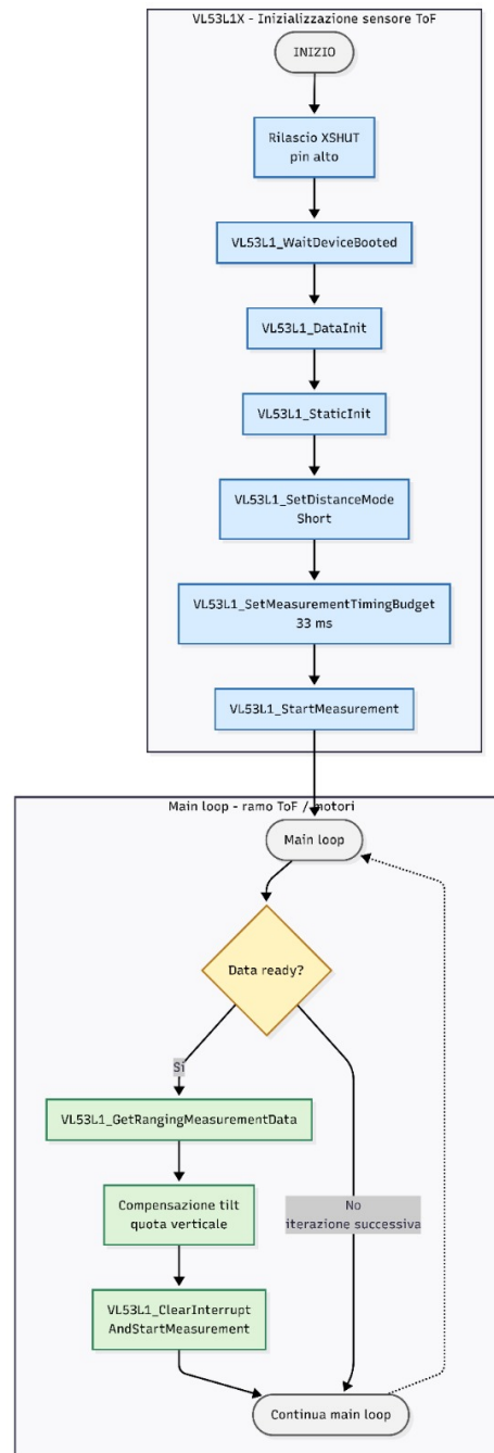
Figura 3.1: Diagramma di flusso del sensore VL53L1X
