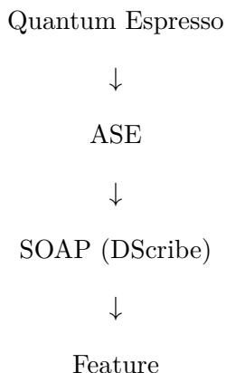
Schema 1.1: Struttura schematica del processo di creazione dei feature vector
