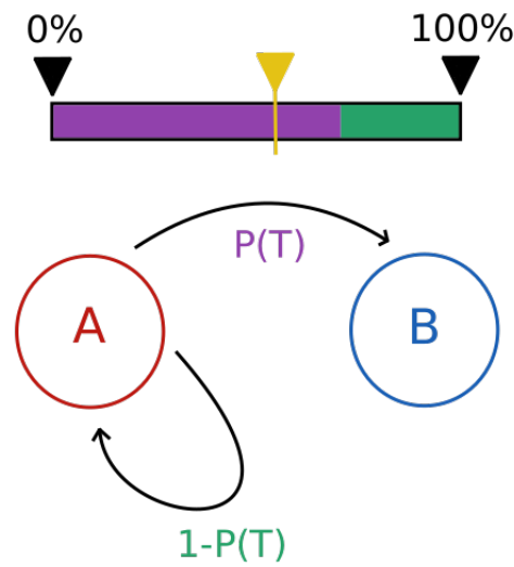
Schema 1.4: Struttura schematica dell'algoritmo di Metropolis
