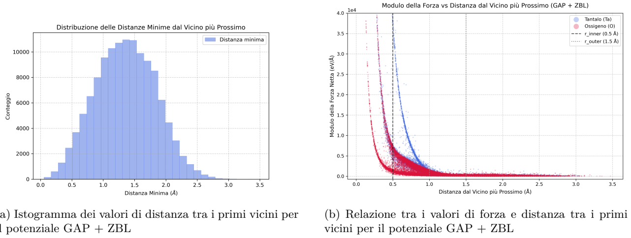
Figura 4.10: Distanze e relazione forze distanze per il potenziale GAP + ZBL, originariamente la scala del pannello (b) raggiungeva 10^7 , è stata modificata in modo da evidenziare la regione di interesse.
