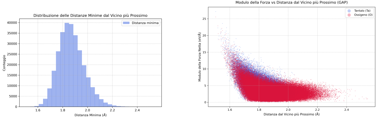
(a) Istogramma dei valori di distanza tra i primi vicini per il set di dati di training
