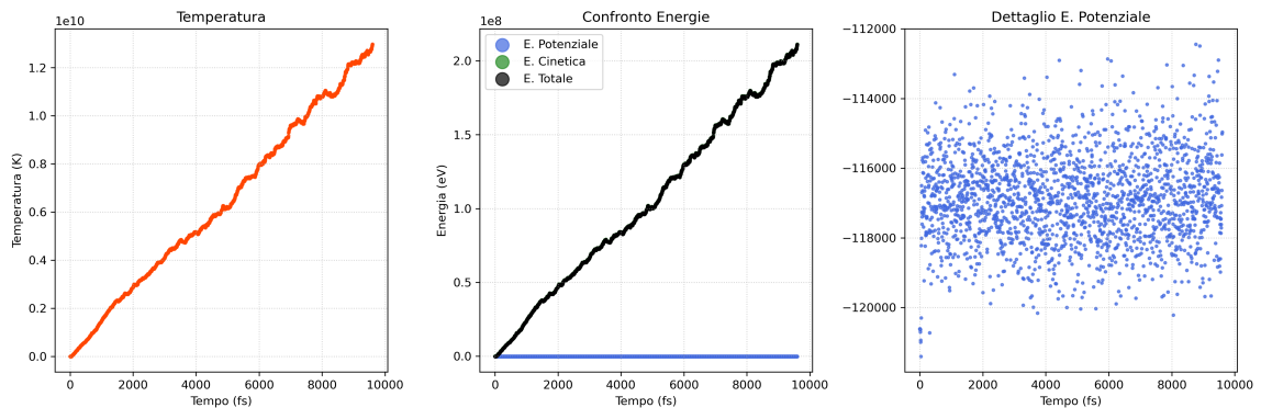
Figura 4.3: Grafico dell'andamento temporale per i valori di energia e temperatura
