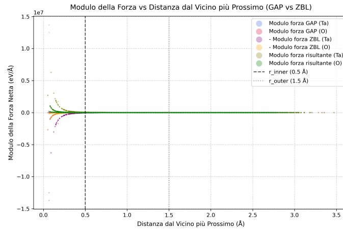
Figura 4.11: Grafico del confronto tra i contributi di forza di GAP e di ZBL
