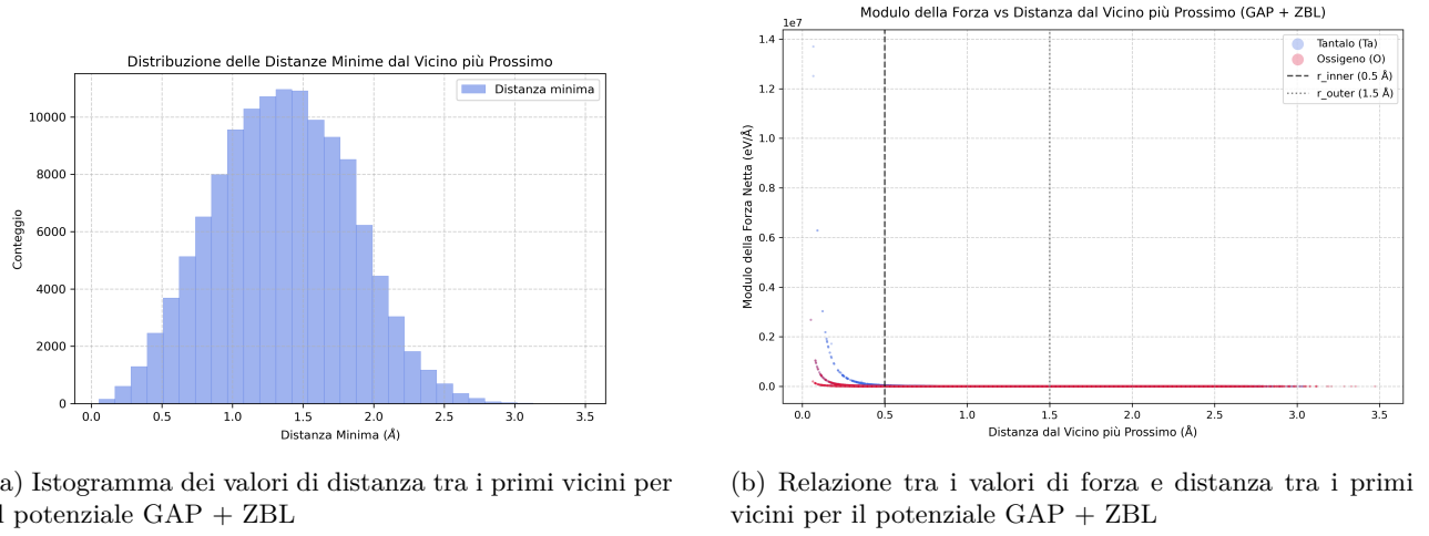
Figura 4.10: Distanze e relazione forze distanze per il potenziale GAP + ZBL.
