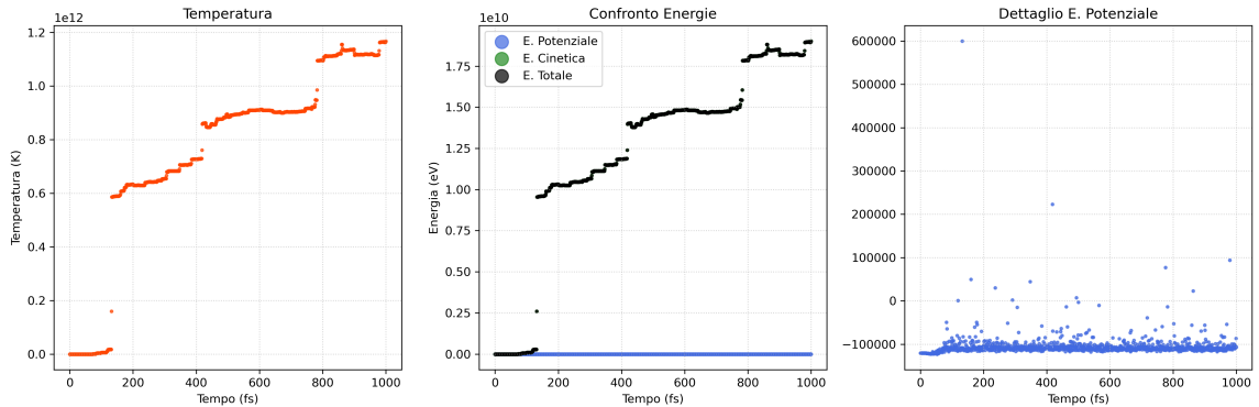
Figura 4.9: Grafico dell'andamento temporale per i valori di energia e temperatura, potenziale GAP + ZBL
