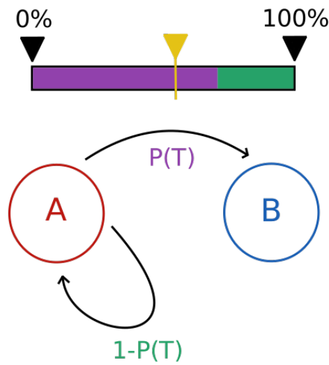
Schema 1.4: Struttura schematica dell'algoritmo di Metropolis
