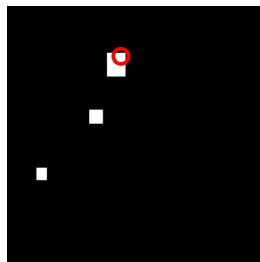
(d) Ours
