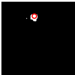
(b) FCN
