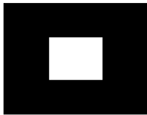
(d) Ours
