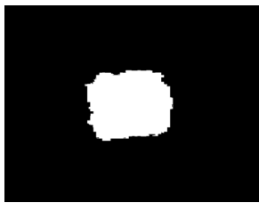
(b) FCN
