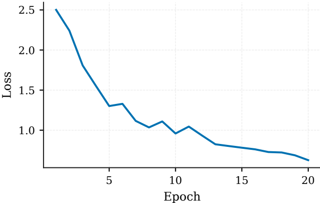
mAP@0.5
