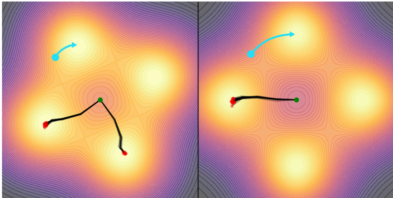
DPPO
