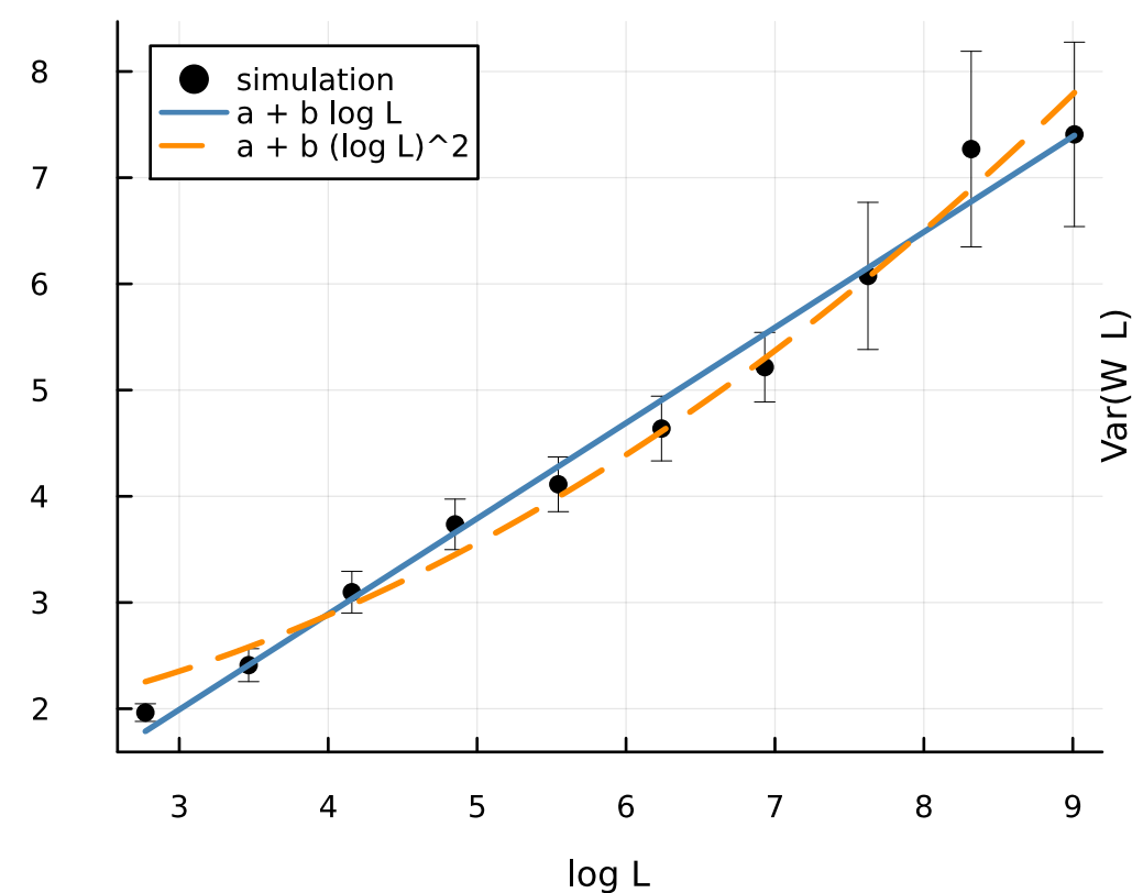
lognormal (sigma=1.0)
