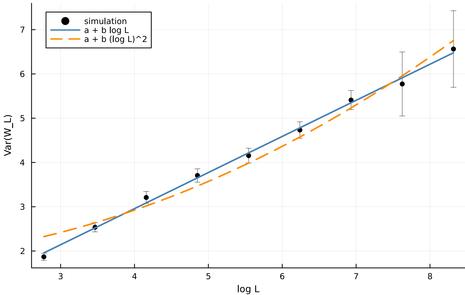
lognormal (sigma=1.0)
