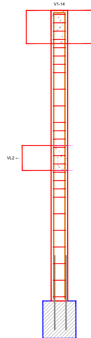
P18 – 30 x 20 (cara de 20, mirando al este)
