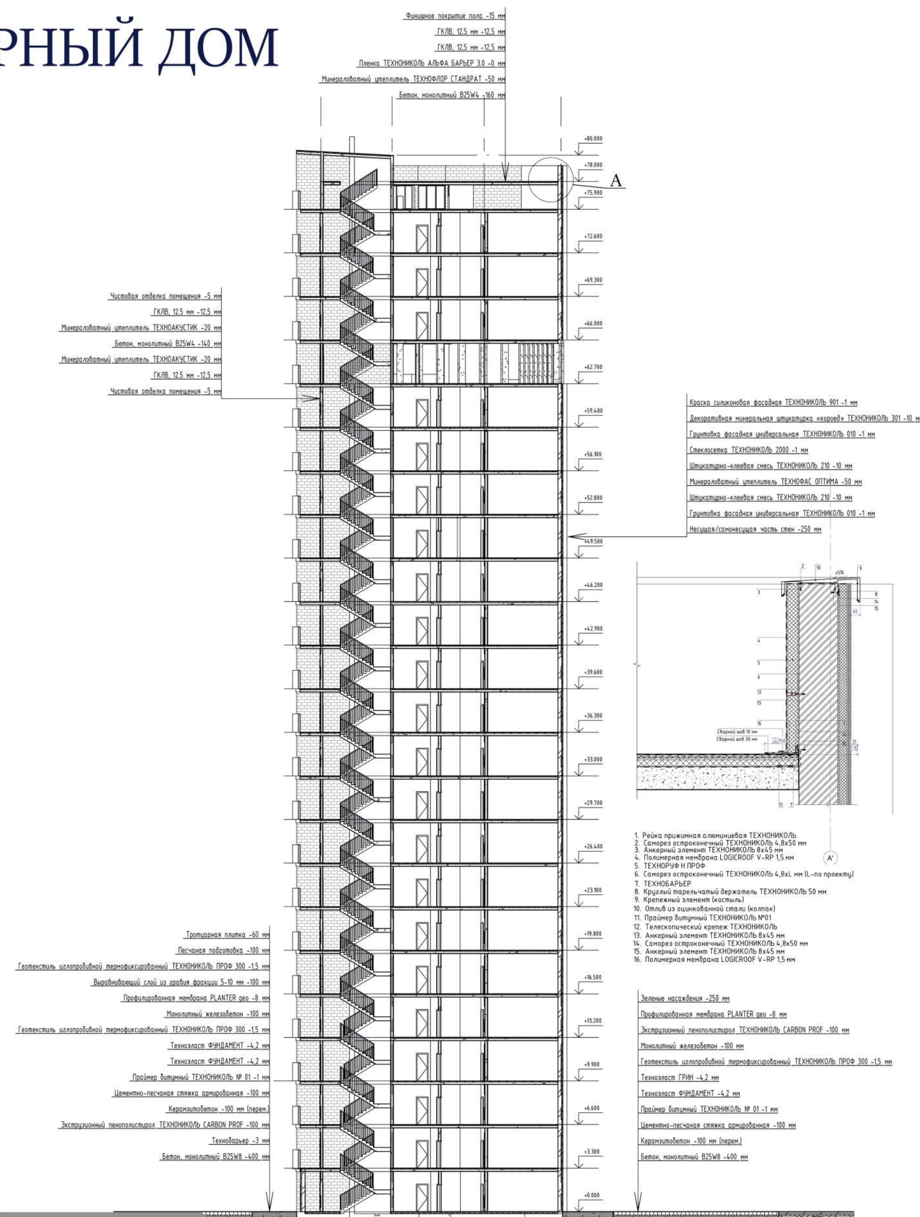
Разрез 1-1 М1:300
