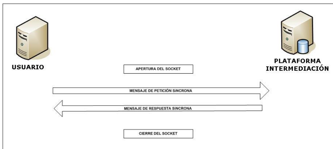
Figura 2.- Esquema comunicaciones peticiones síncronas
