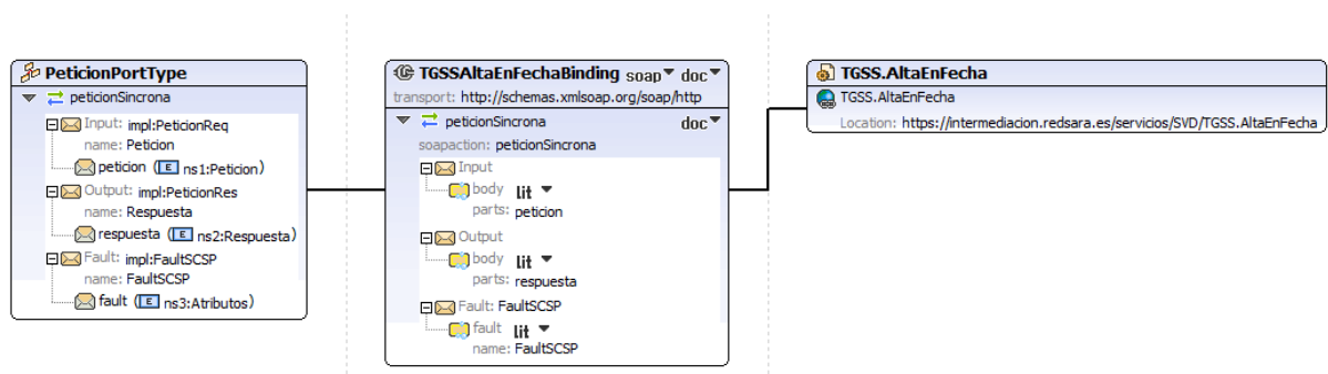
Figura 3.- Diagrama de la Interfaz WSDL del servicio síncrono
