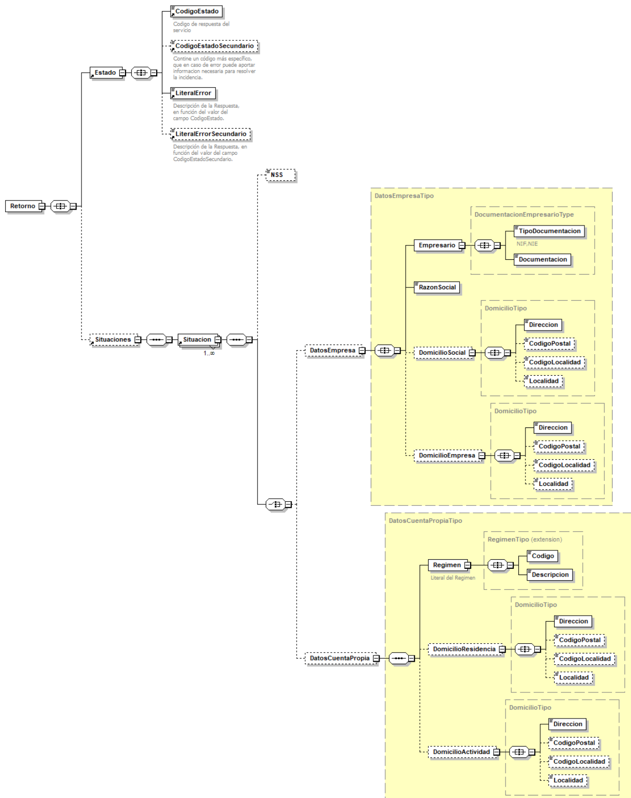
Figura 11.- Diagrama Datos Específicos de la etiqueta &lt;Retorno&gt;
