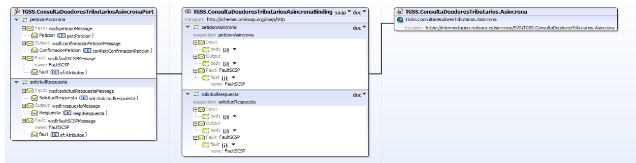
Figura 5.- Diagrama de la Interfaz WSDL del servicio asíncrono
