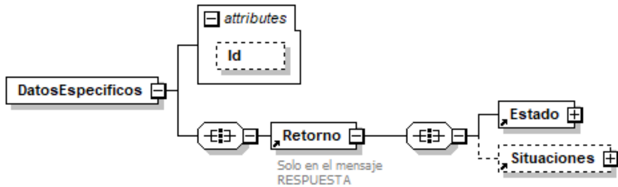
Figura 10.- Diagrama de Datos Específicos de la Respuesta
