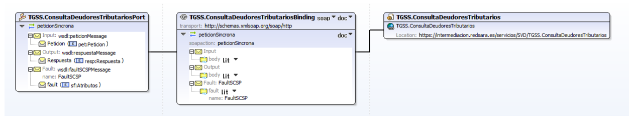
Figura 4.- Diagrama de la Interfaz WSDL del servicio síncrono
