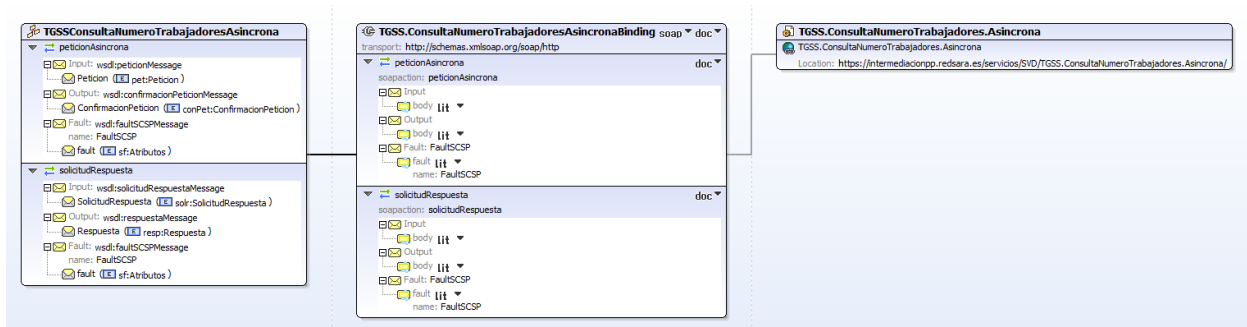
Figura 4.- Diagrama de la Interfaz WSDL del servicio asíncrono
