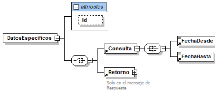
Figura 9.- Diagrama de Datos Específicos de la Petición
