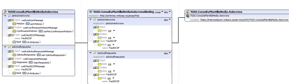
Figura 3.- Diagrama de la Interfaz WSDL del servicio asíncrono
