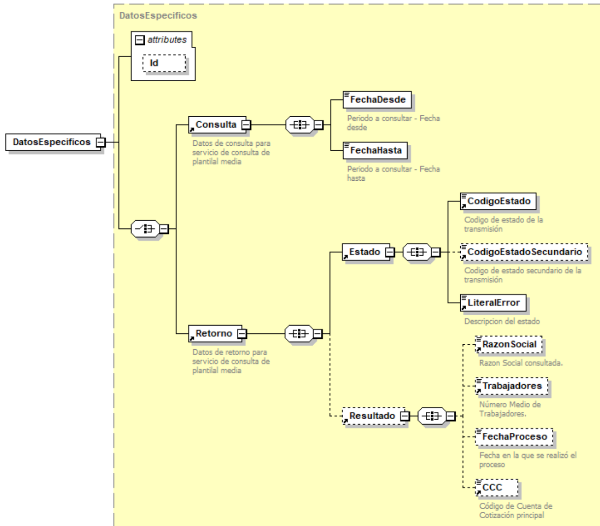
Figura 8.- Diagrama de Datos Específicos del Servicio
