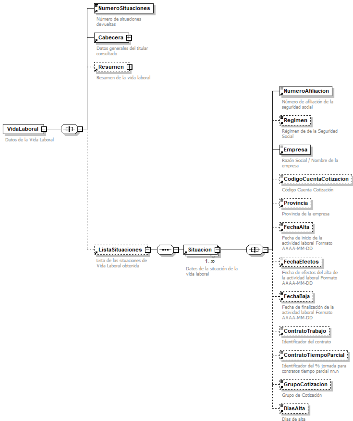
Figura 12.- Diagrama del tag <ListaSituaciones> de <VidaLaboral>
