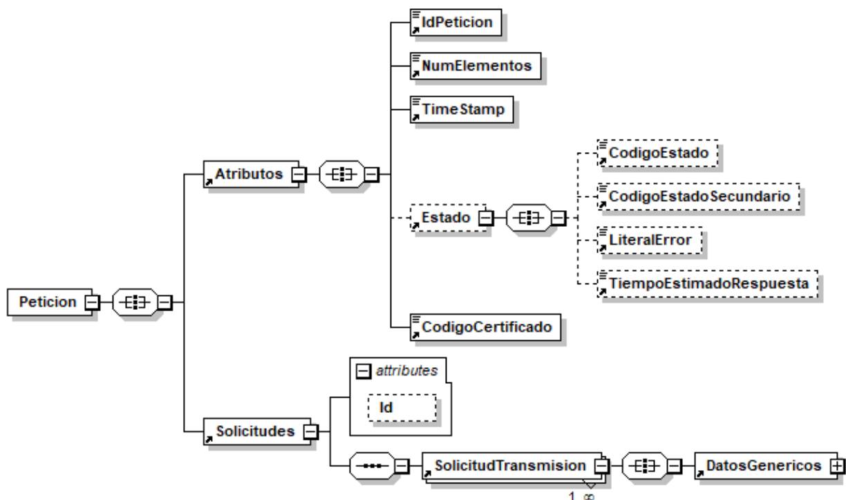
Figura 6.- Diagrama del mensaje de petición del servicio
