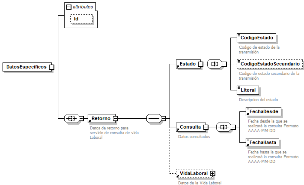
Figura 10.- Diagrama de datos específicos del servicio
