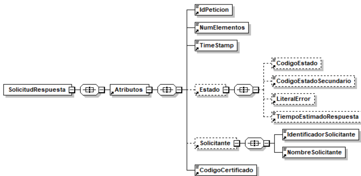
Figura 14.- Diagrama del mensaje de solicitud de respuesta del servicio
