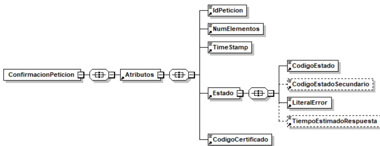
Figura 13.- Diagrama del mensaje de confirmación de petición del servicio
