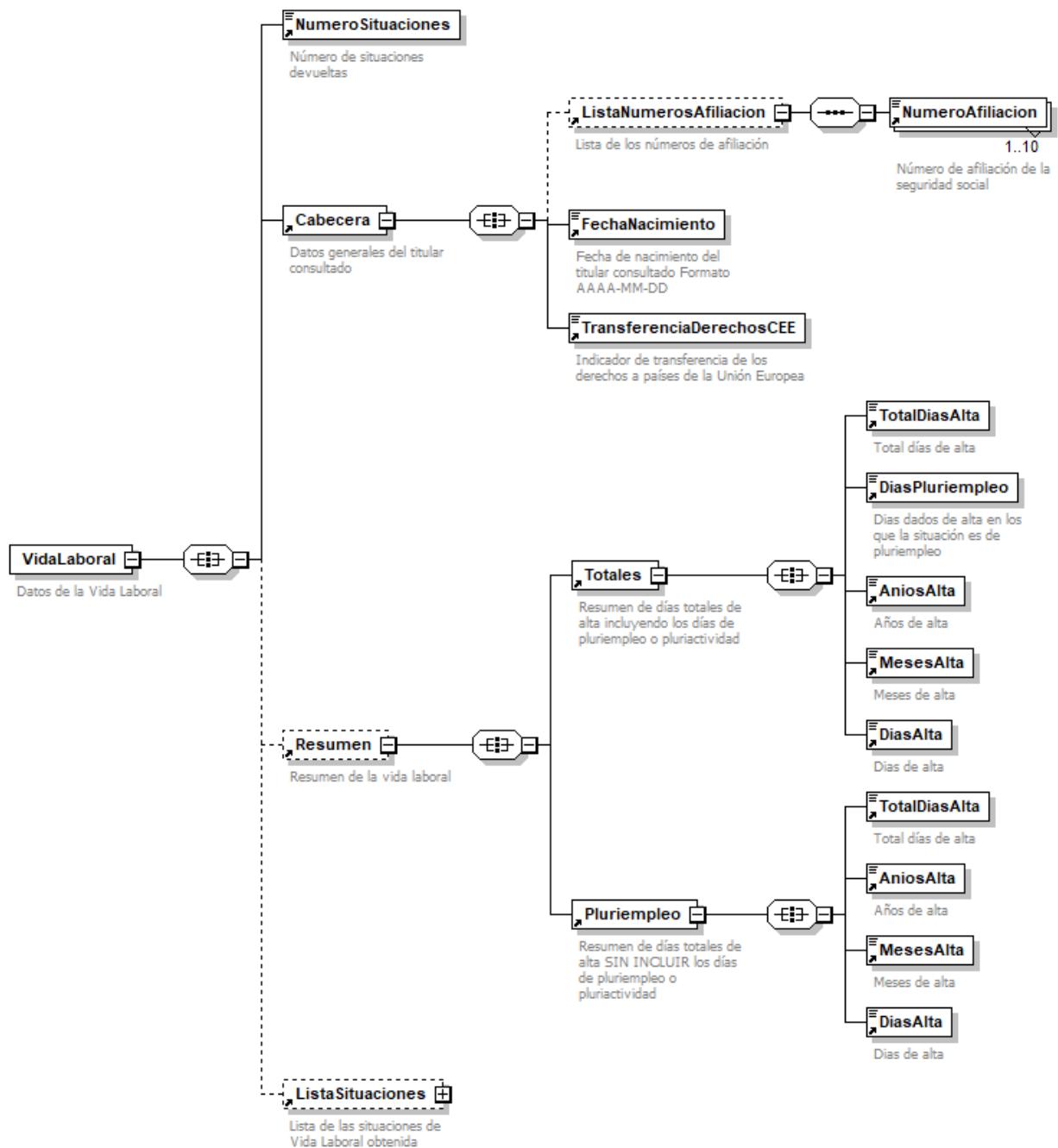
Figura 11.- Diagrama del tag <VidaLaboral> de datos específicos
