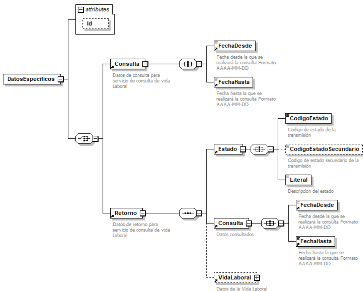
Figura 10.- Diagrama de datos específicos del servicio
