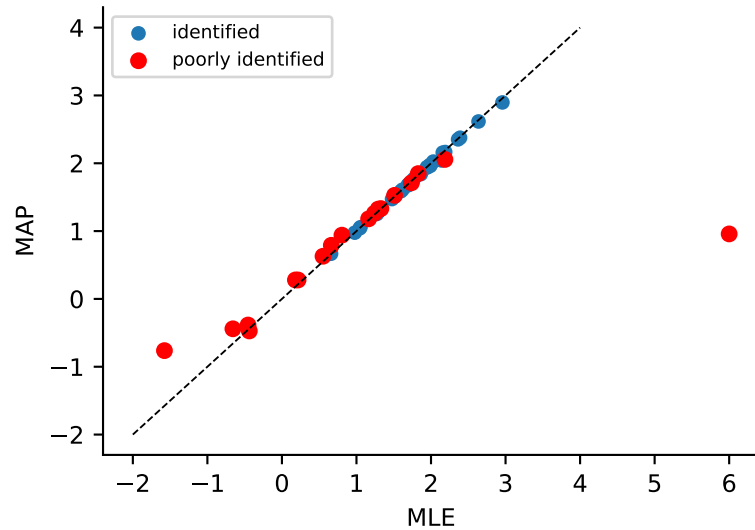
\log \beta : r=0.999
