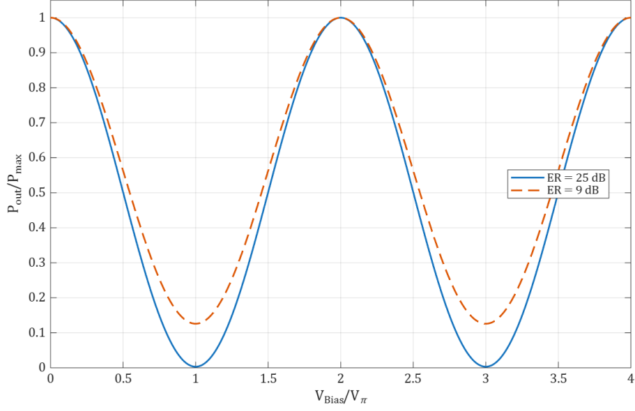
Figura 13 – Potencia de salida normalizada para ER = 25 dB y ER = 9 dB.
