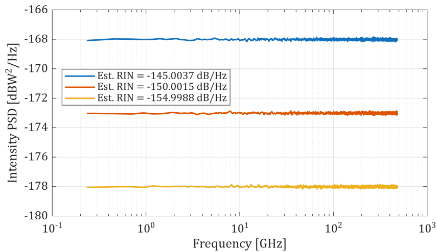
Figura 2 – Densidad espectral de potencia de las fluctuaciones de intensidad para los tres valores de RIN.
