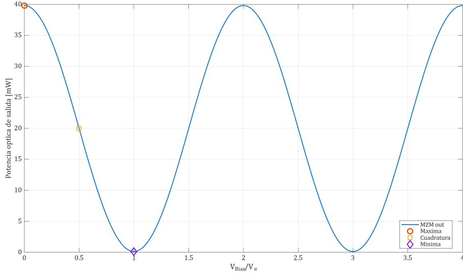
Figura 11 – Potencia óptica de salida del MZM con ER = 25 dB e IL = 4 dB.
