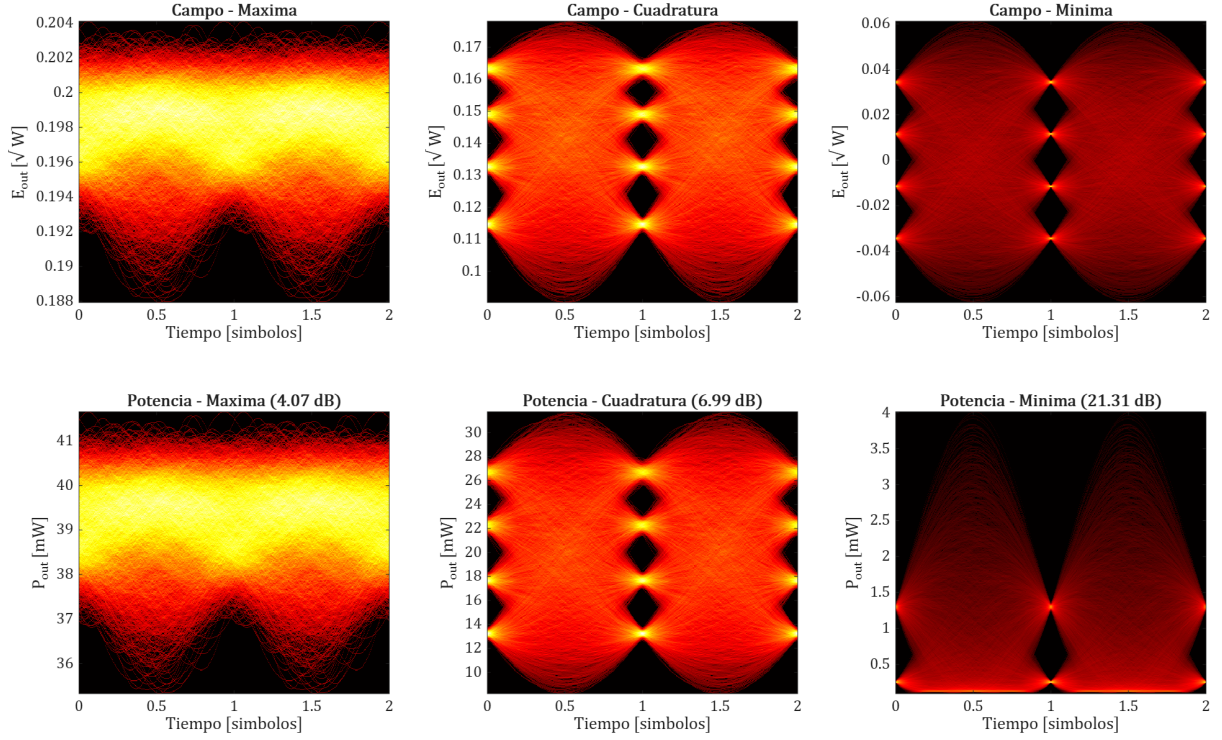
Figura 16 – Diagramas de ojo a la salida del MZM: campo eléctrico (arriba) y potencia óptica (abajo) en máxima, cuadratura y mínima.
