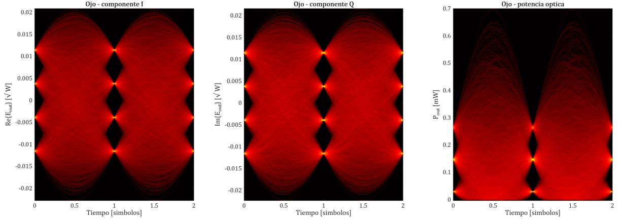
Figura 18 – Diagramas de ojo a la salida del MZM-IQ: componente I, componente Q y potencia óptica.
