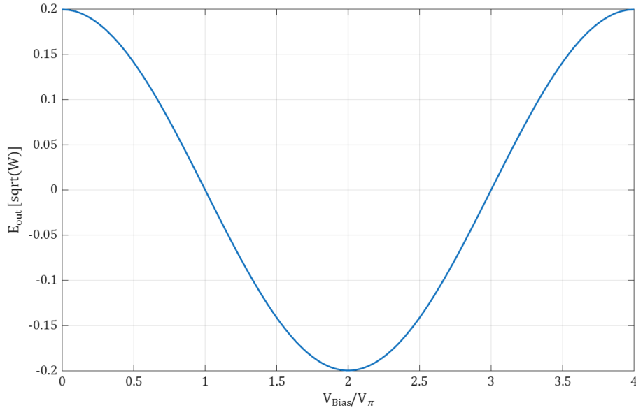
Figura 12 – Campo eléctrico de salida del MZM con ER = 25 dB e IL = 4 dB.
