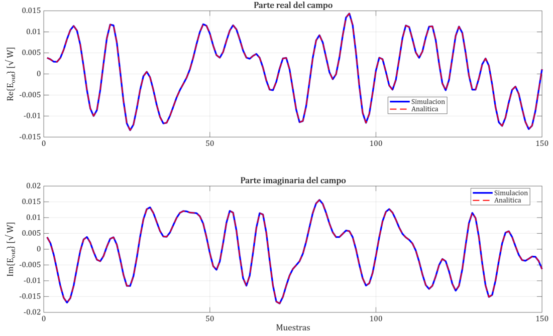
Figura 17 – Partes real e imaginaria del campo de salida del MZM-IQ: simulación y expresión analítica.
