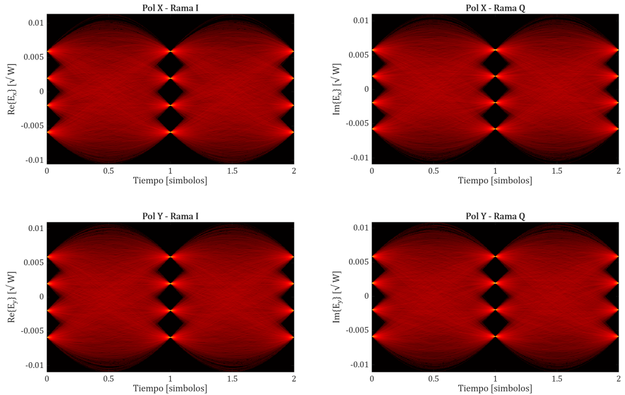
Figura 20 – Diagramas de ojo de las ramas I y Q de las polarizaciones x e y del modulador DP-IQ.
