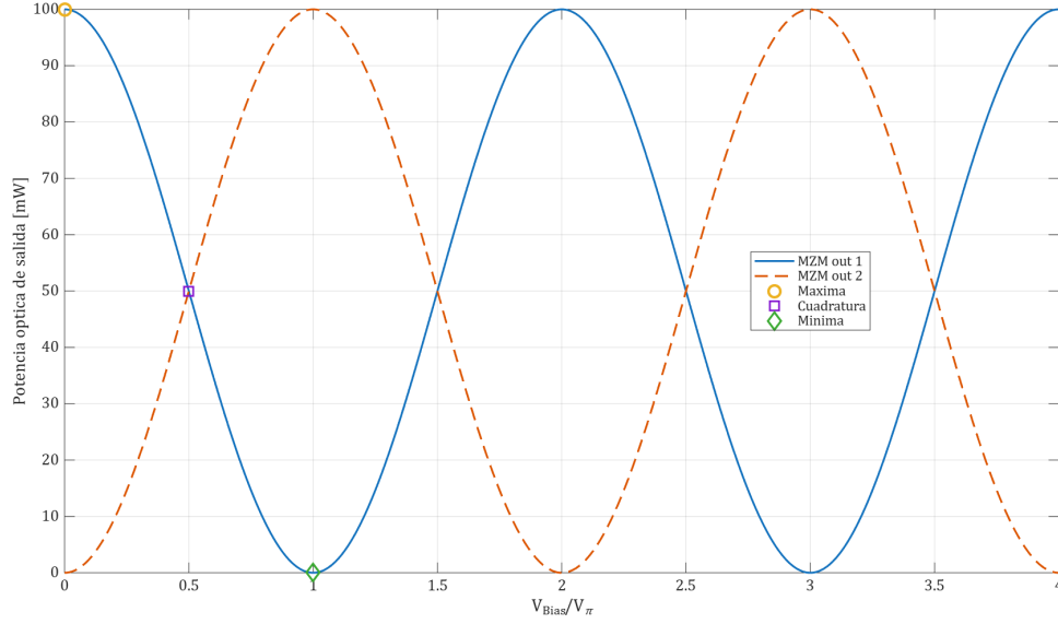
Figura 7 – Potencia óptica en los dos puertos de salida del MZM en función de V_{Bias}/V_{\pi} , con los puntos de máxima, cuadratura y mínima.
