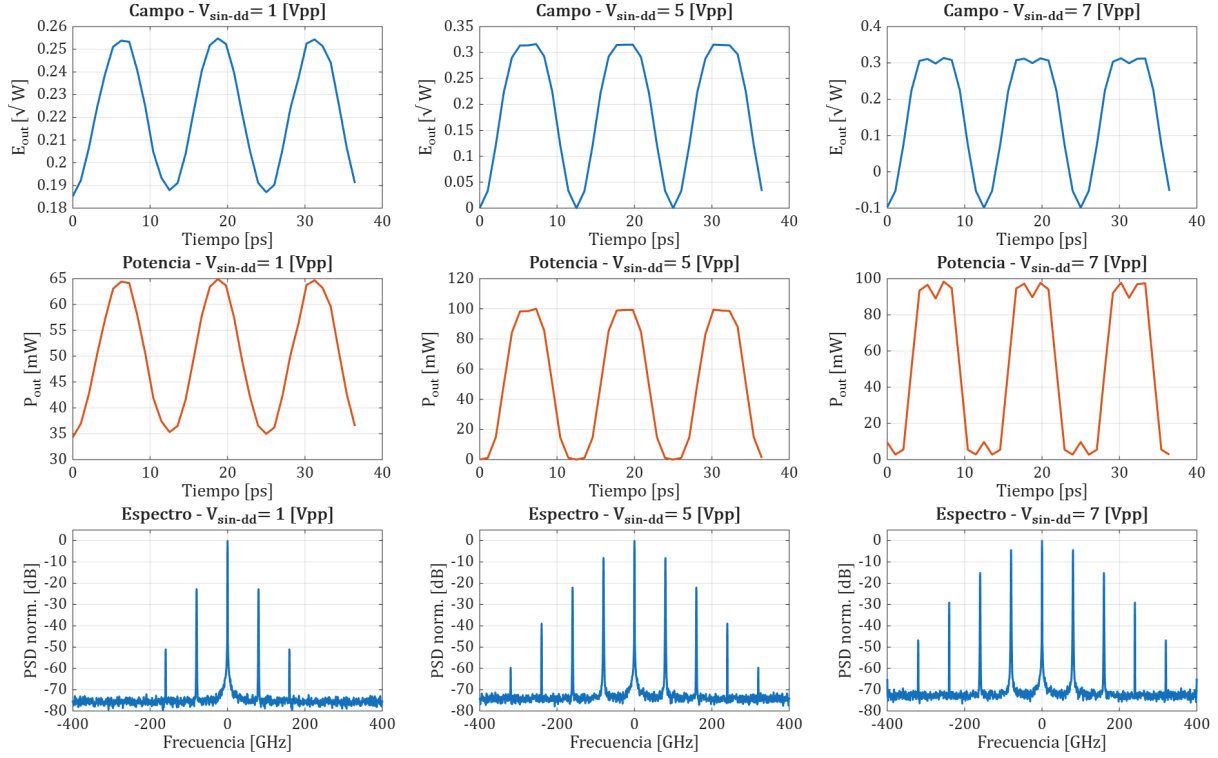
Figura 9 – Campo eléctrico (arriba), potencia óptica (centro) y espectro del campo (abajo) con el MZM polarizado en cuadratura.
