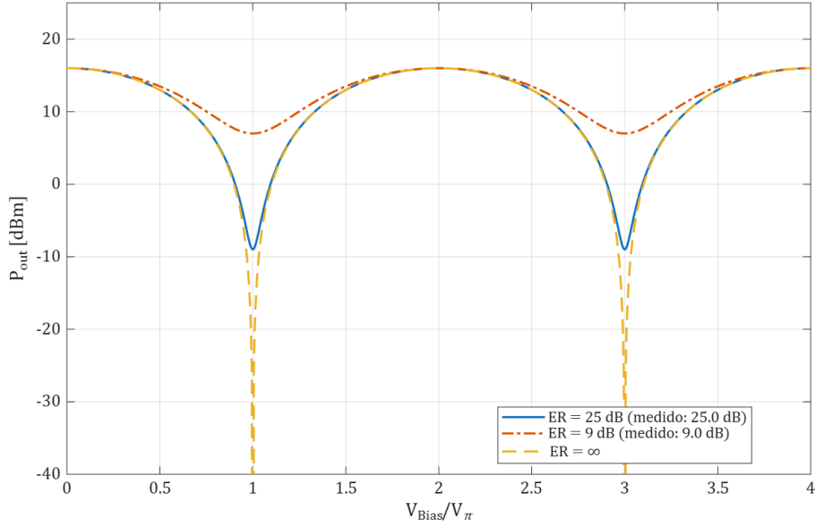
Figura 14 – Potencia de salida en dBm para ER = 25 dB, ER = 9 dB y para el MZM ideal ( ER = \infty ), con IL = 4 dB.
