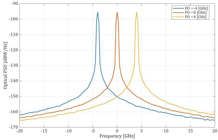
Figura 3 – Densidad espectral óptica para los tres valores de offset de frecuencia.
