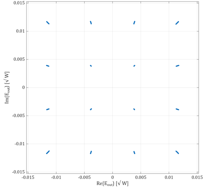
Figura 19 – Constelación a la salida del MZM-IQ en los instantes de muestreo.
