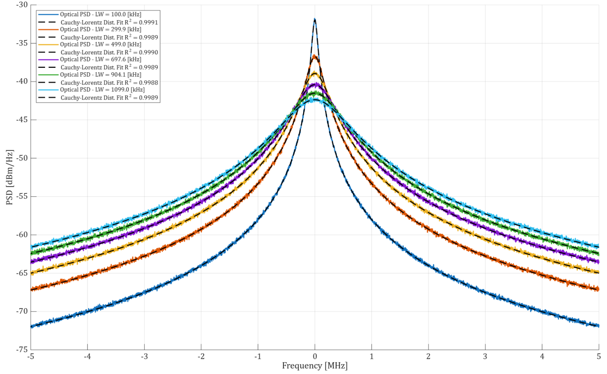
Figura 4 – Densidad espectral óptica simulada (color) y ajuste de Cauchy-Lorentz (línea punteada) para cada ancho de línea.
