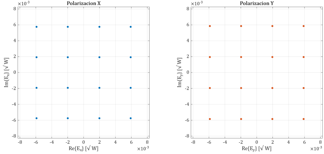
Figura 21 – Constelación 16-QAM en cada polarización del modulador DP-IQ.
