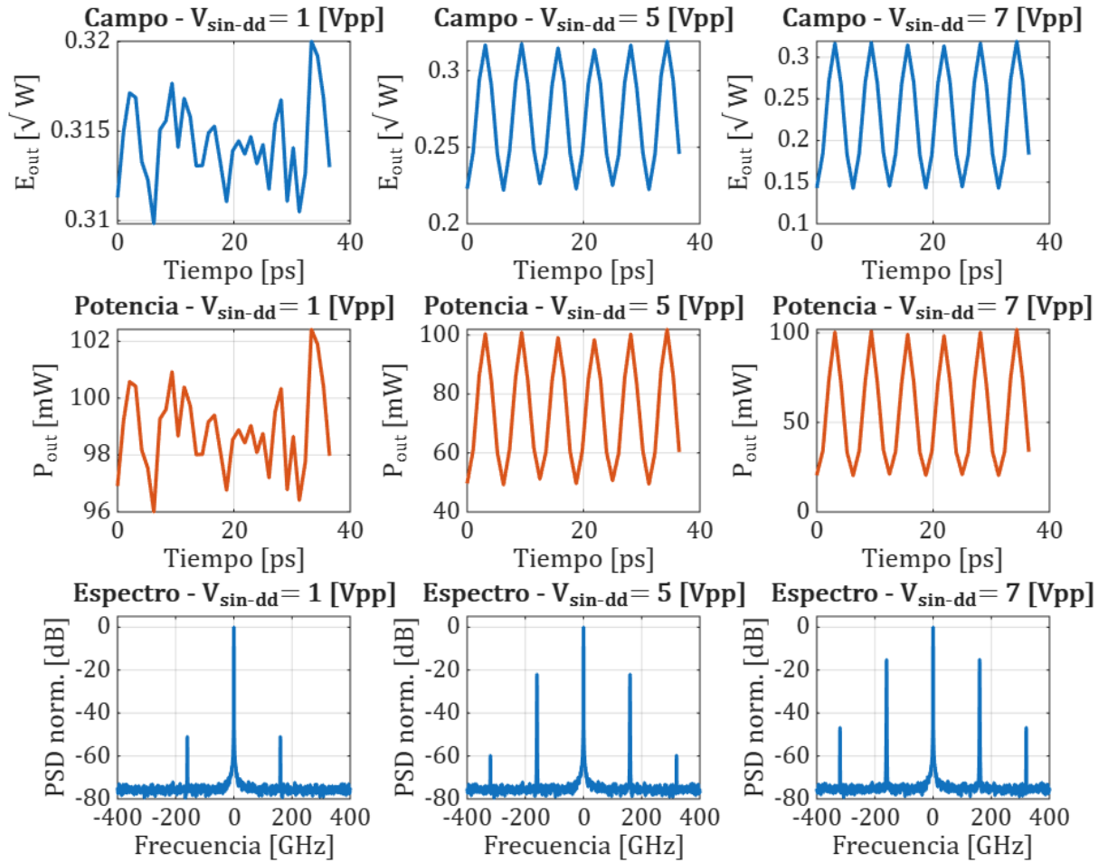
Figura 8 – Campo eléctrico (arriba), potencia óptica (centro) y espectro del campo (abajo) con el MZM polarizado en máxima.
