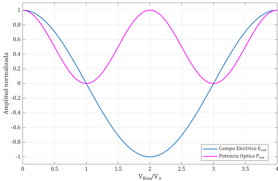
Figura 6 – Campo eléctrico y potencia óptica normalizados a la salida del MZM ideal en función de la tensión de polarización.
