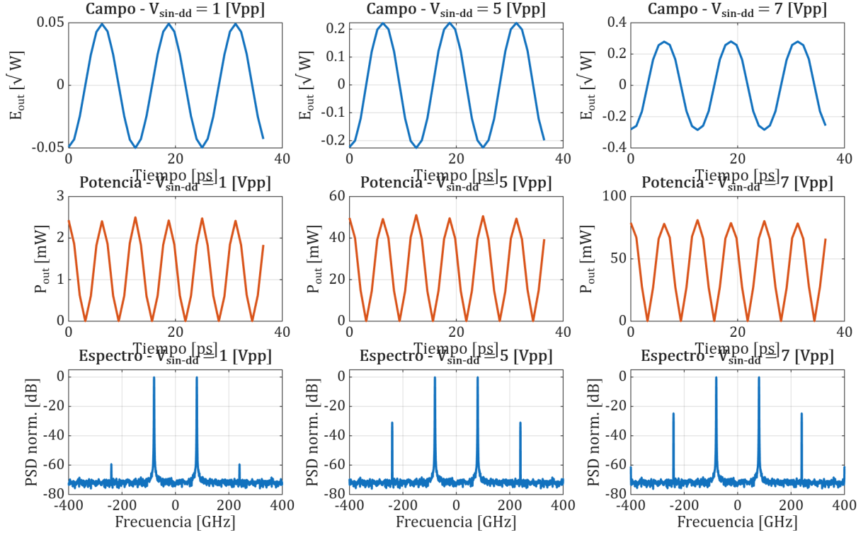
Figura 10 – Campo eléctrico (arriba), potencia óptica (centro) y espectro del campo (abajo) con el MZM polarizado en mínima.
