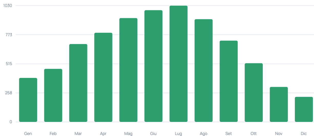
PRODUZIONE MENSILE (KWH) - PROFILO ANNUALE
