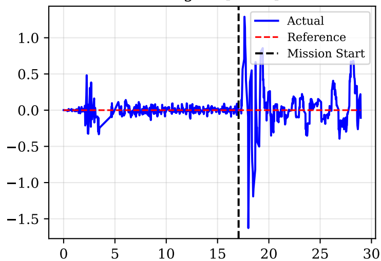
Omega Y [rad/s]
