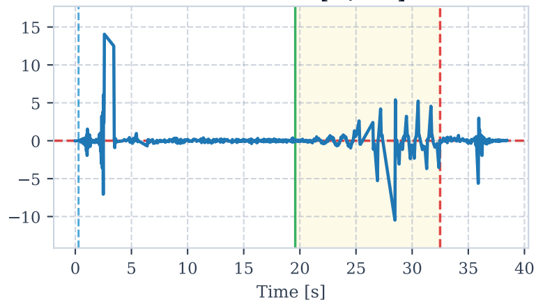
Angular Acc Y [rad/s 2 ]
