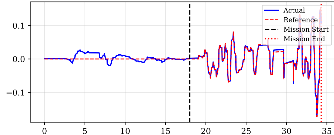
Roll [rad]
